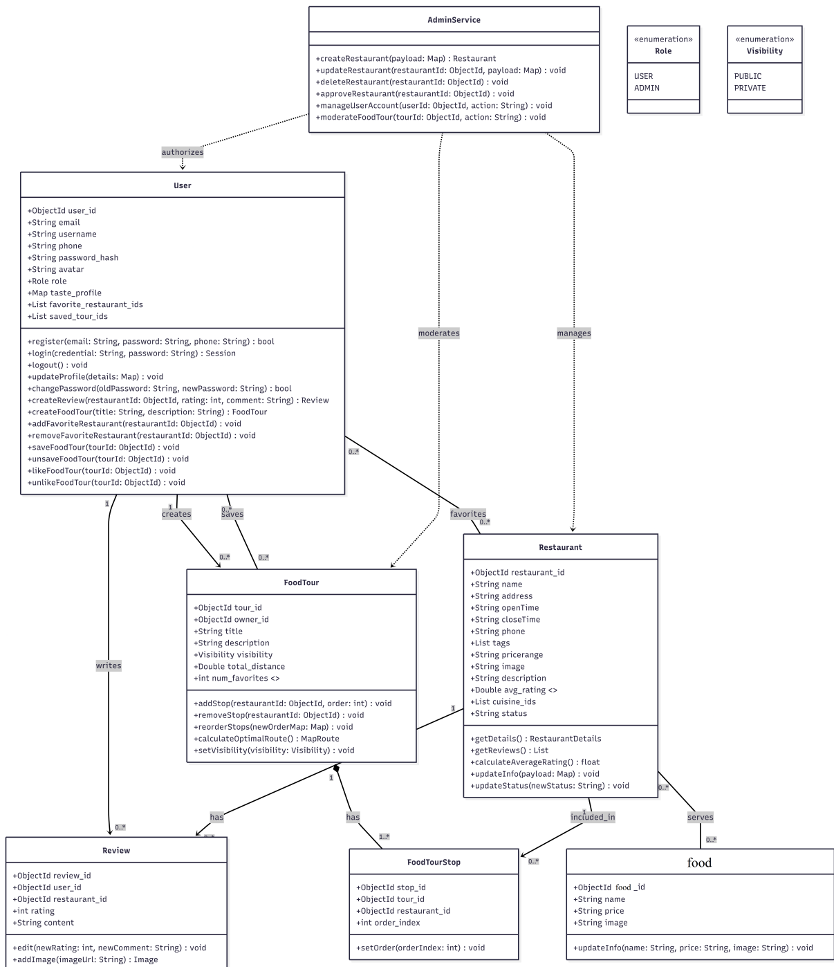
Hình 4.16: Class Diagram
