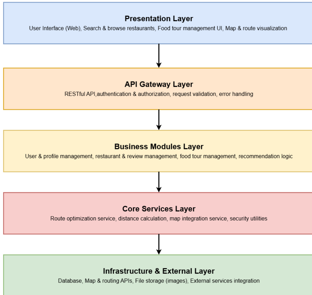
Hình 5.1: Layered Architecture
