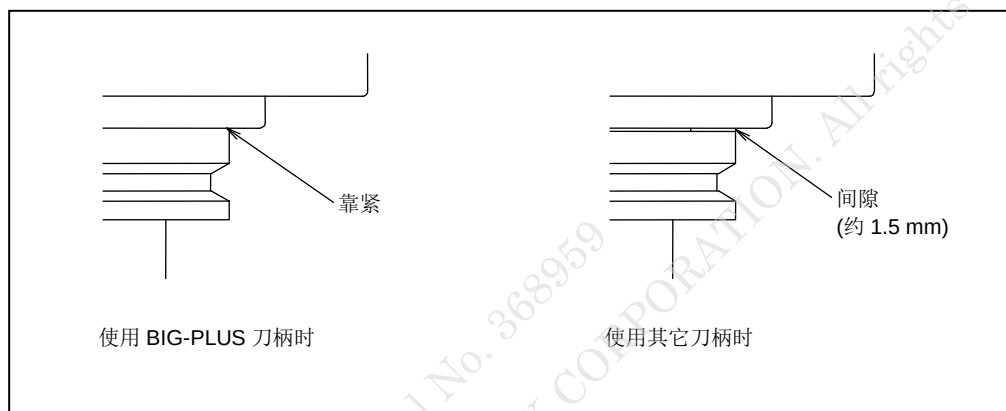
Fig. 2-1 安装刀柄时产生的间隙
