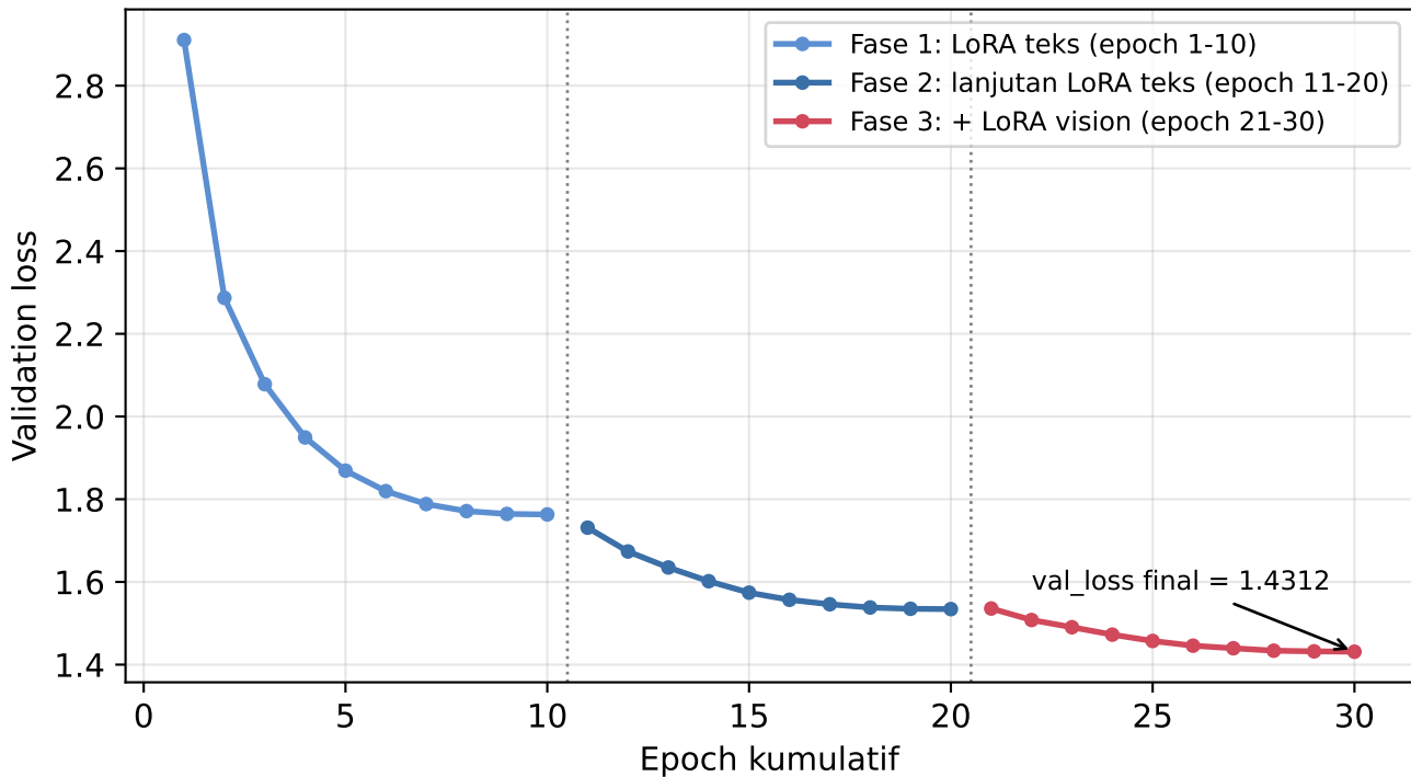
Konvergensi training BLIP (30 epoch, 3 fase)
