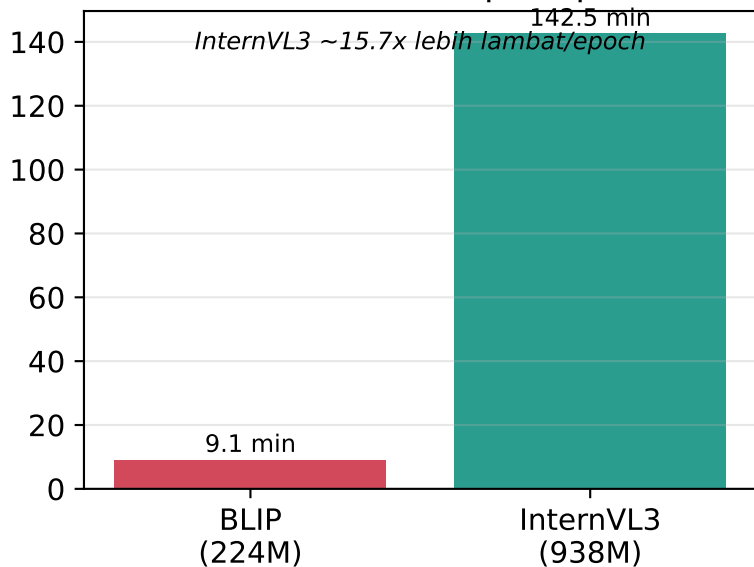
Waktu wall-clock per epoch
