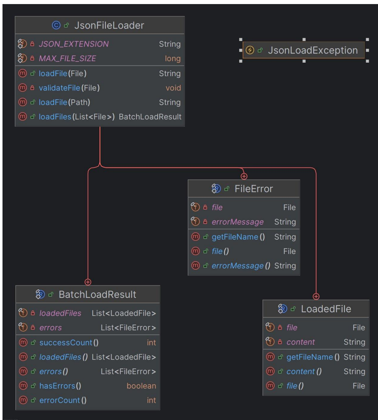
Rysunek 2.4 Diagram klas - pakiet loader
