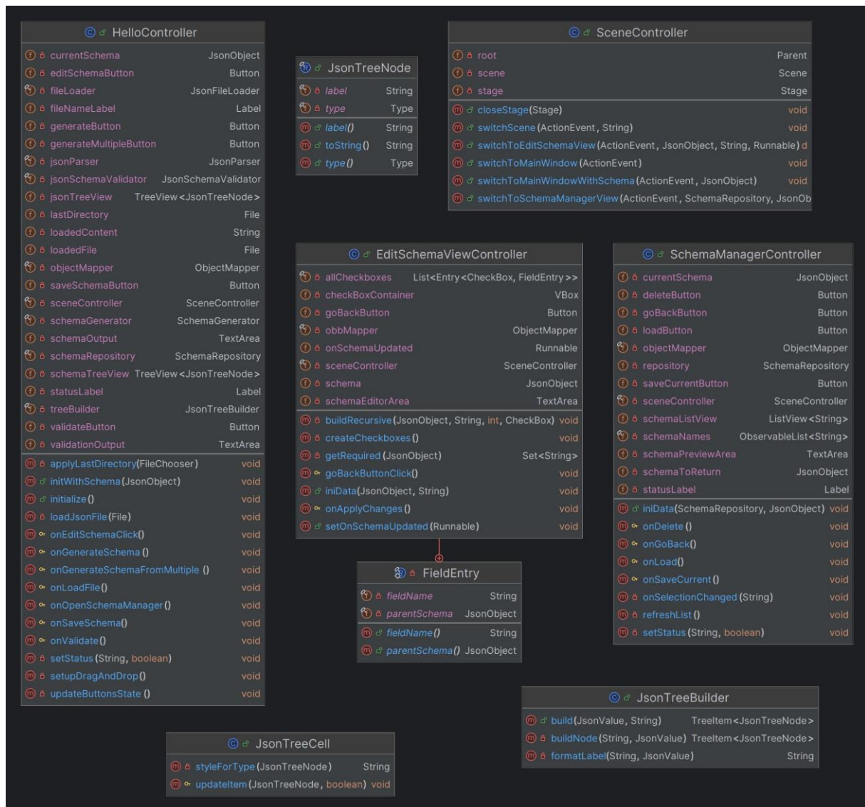
Rysunek 2.7 Diagram klas - warstwa prezentacji
