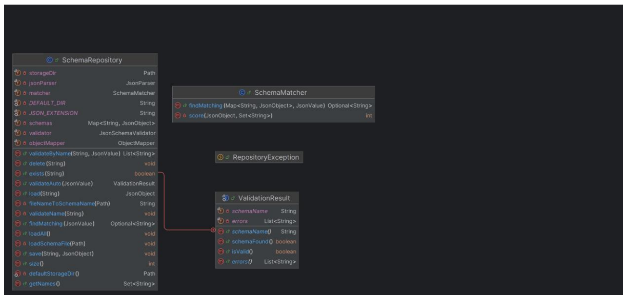
Rysunek 2.6 Diagram klas - pakiet database
