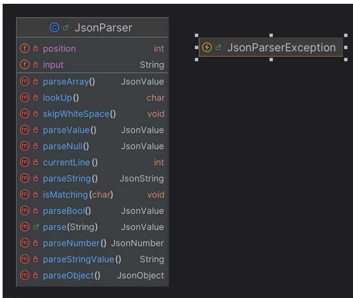
Rysunek 2.3 Diagram klas - pakiet parser
