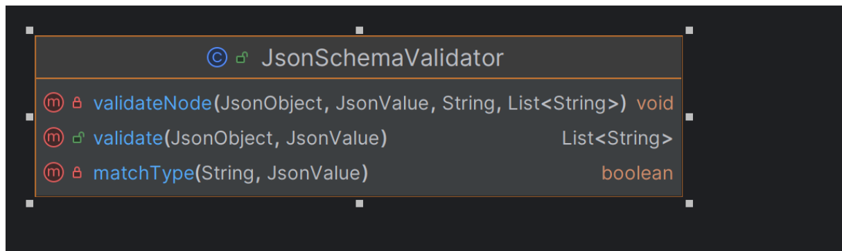
Rysunek 2.5 Diagram klas - pakiet validator
