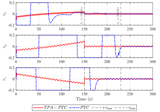
(d) Control torque ( T_f = 150 s)
