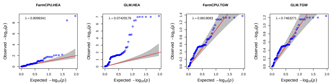
Fig. 3: text
