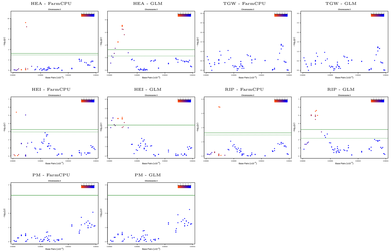
Fig. 4: text
