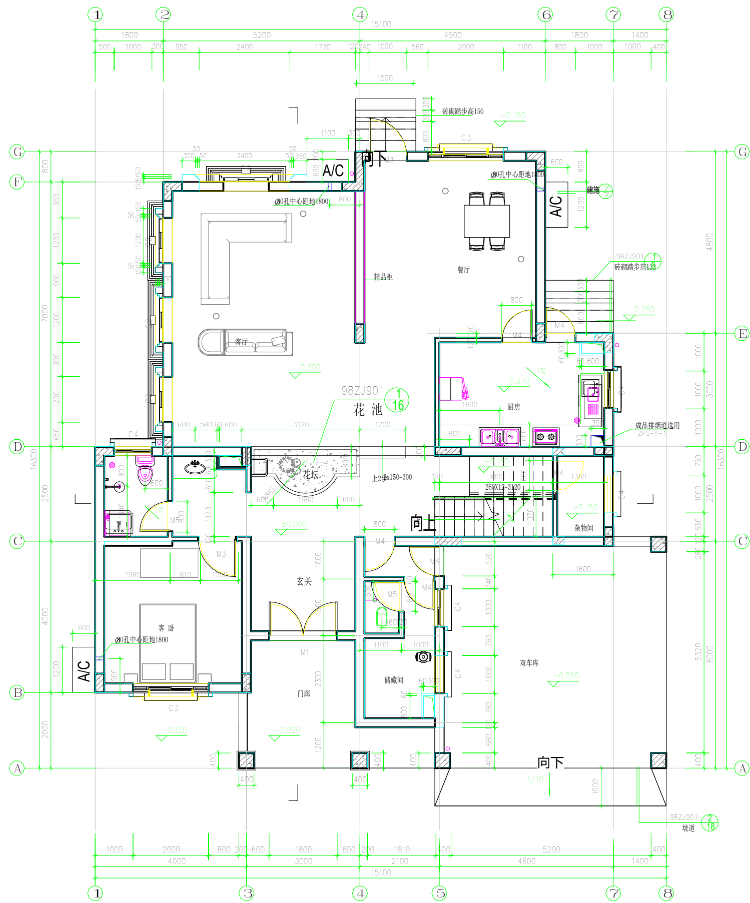
一层平面图 1:50
