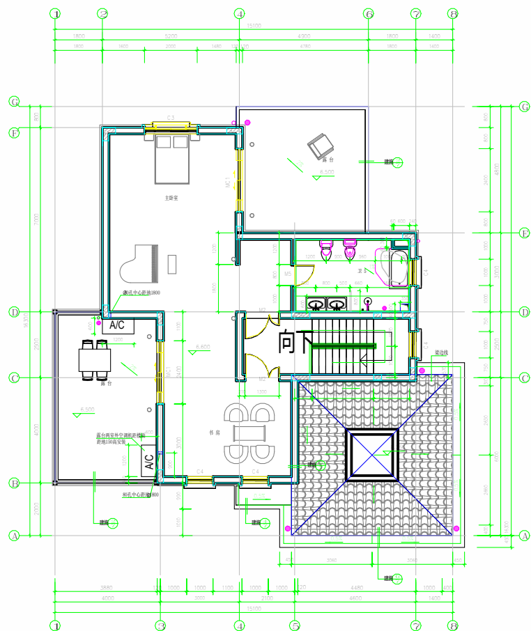
三层平面图 1:50
