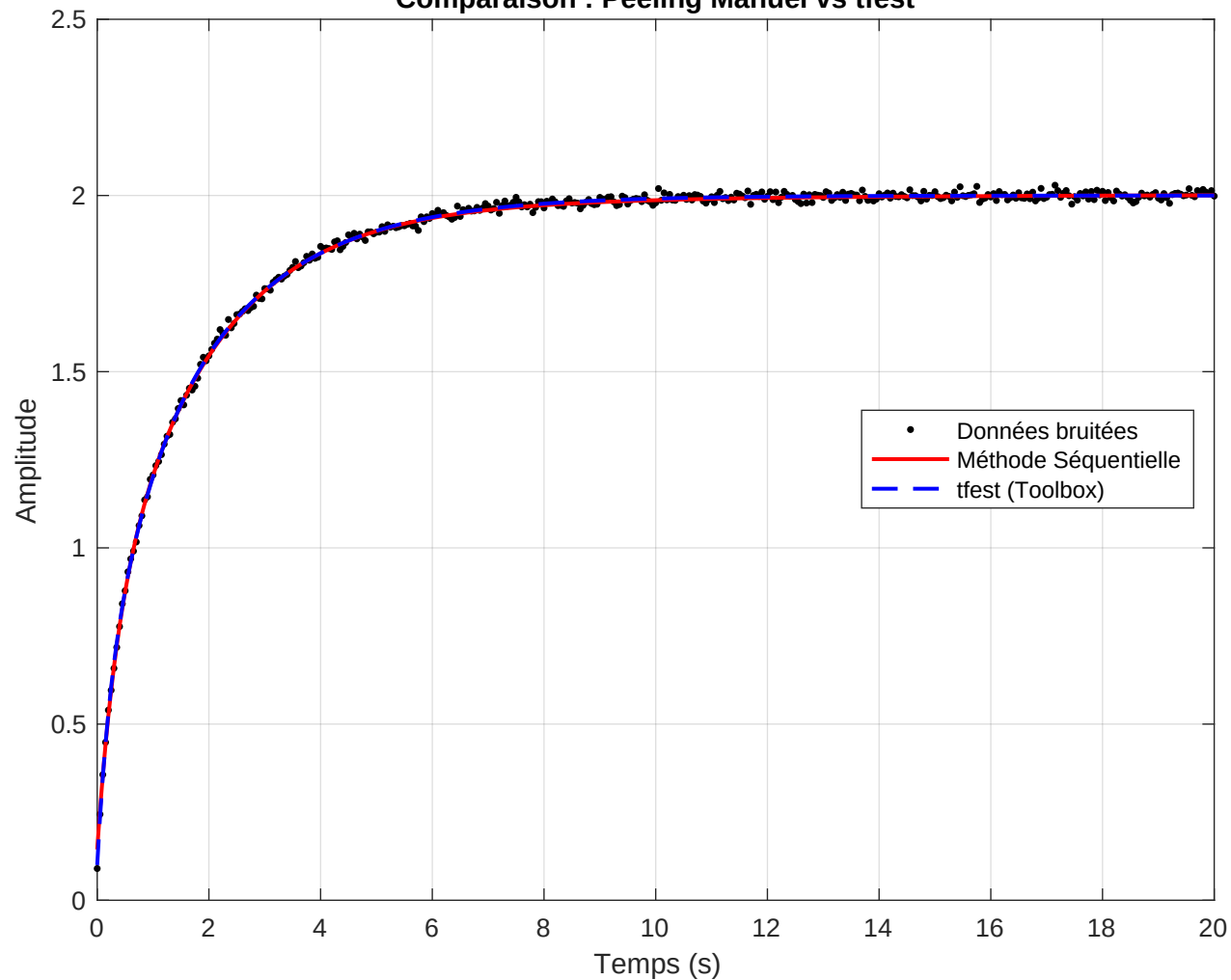
Comparaison : Peeling Manuel vs tfest
