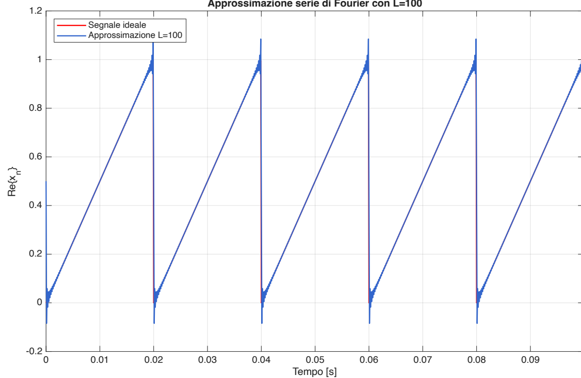
Approssimazione serie di Fourier con L=100
