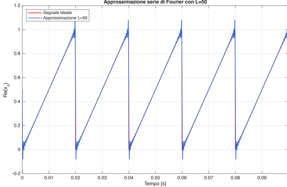
Approssimazione serie di Fourier con L=50
