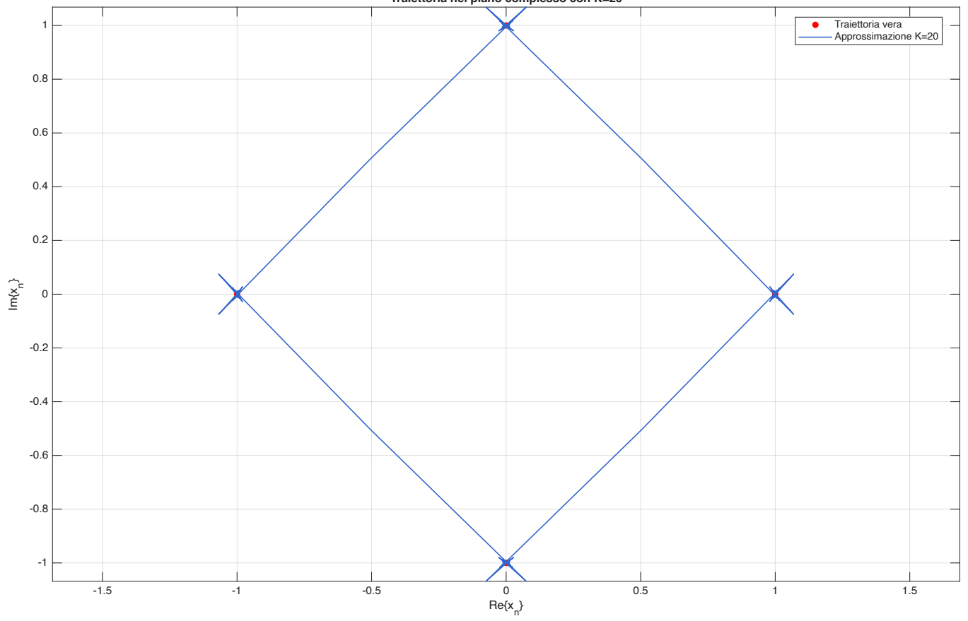
Traiettoria nel piano complesso con K=20
