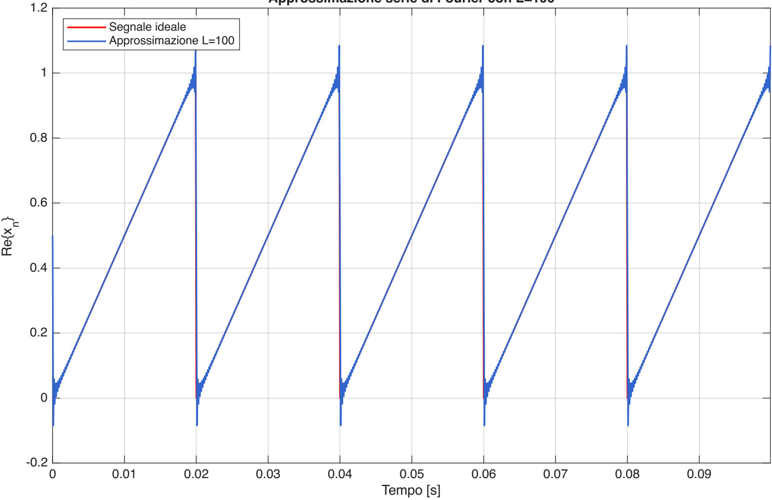
Approssimazione serie di Fourier con L=100
