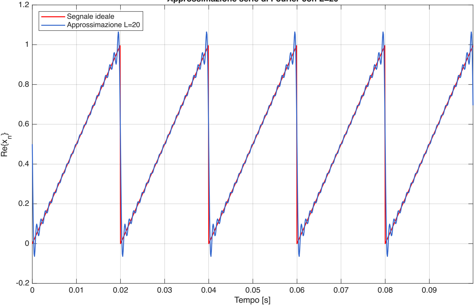
Approssimazione serie di Fourier con L=20
