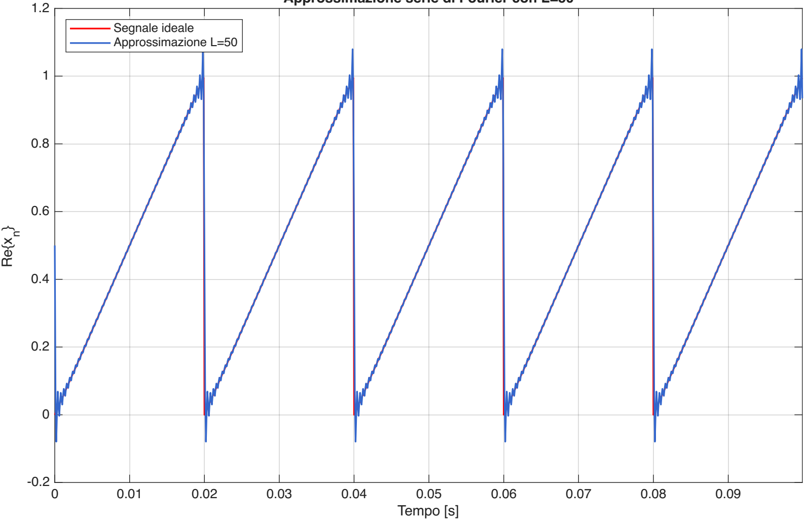
Approssimazione serie di Fourier con L=50
