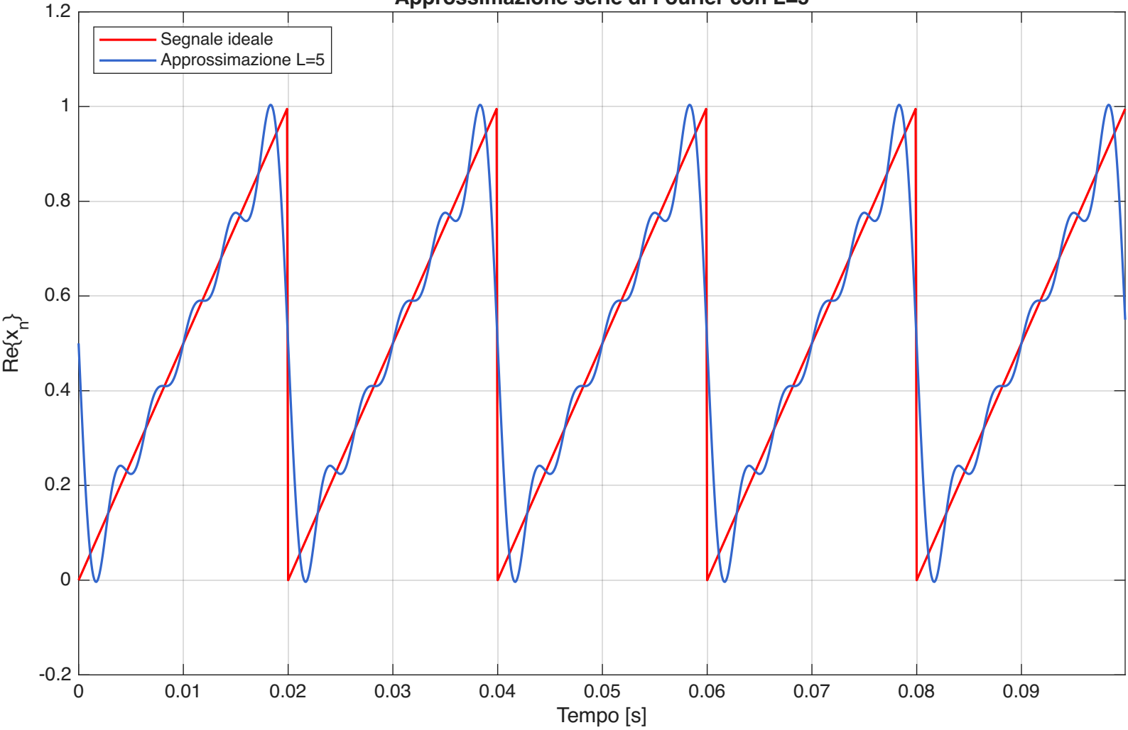
Approssimazione serie di Fourier con L=5
