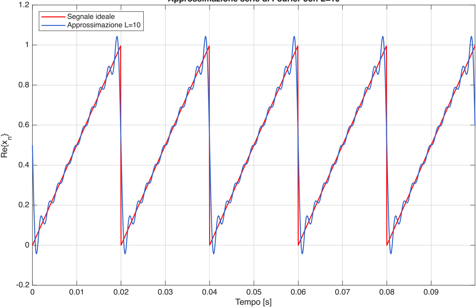
Approssimazione serie di Fourier con L=10
