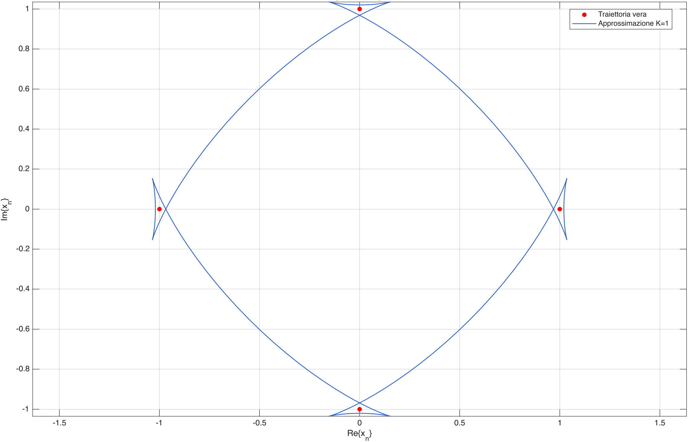
Traiettoria nel piano complesso con K=1
