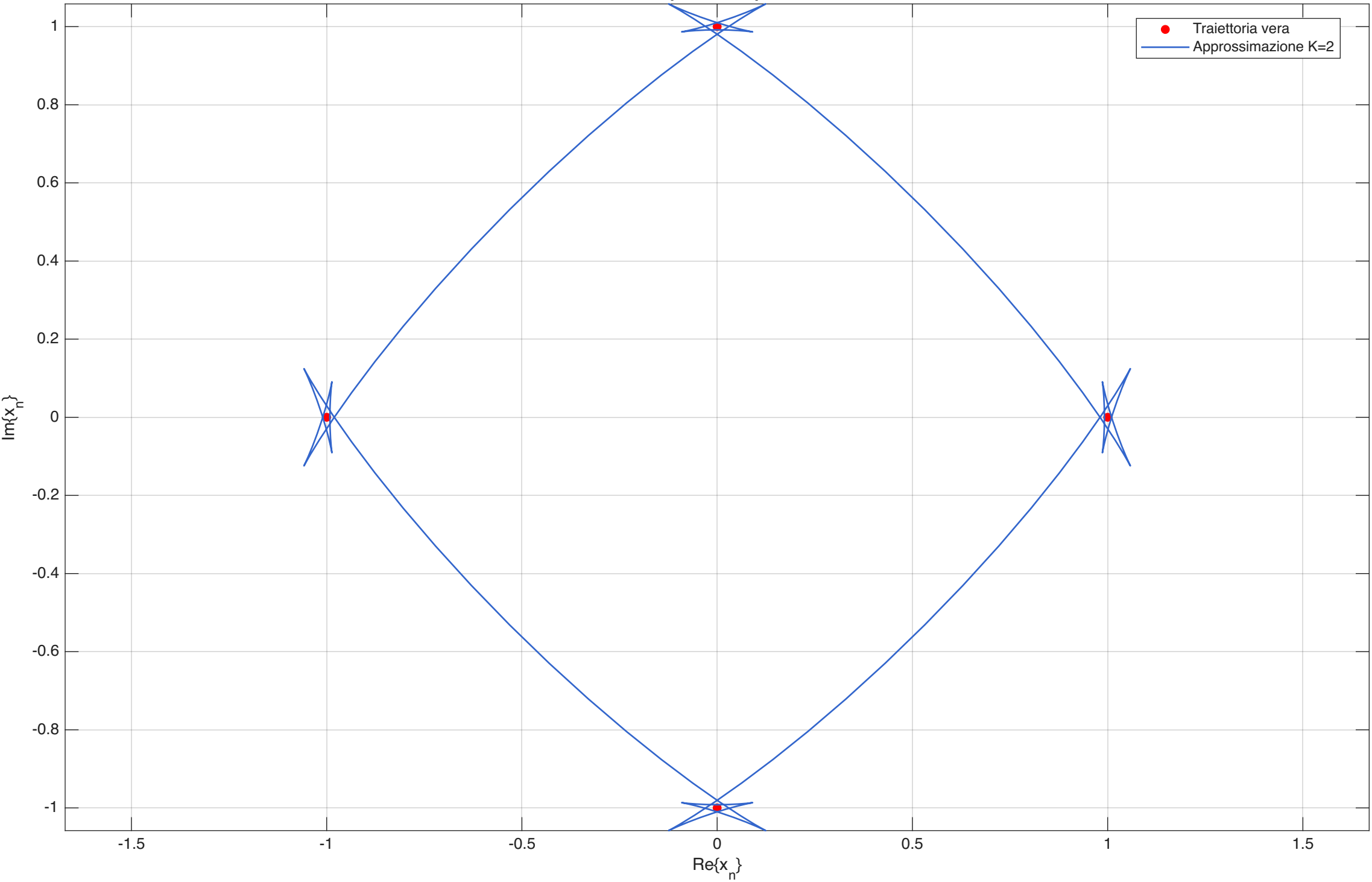
Traiettoria nel piano complesso con K=2
