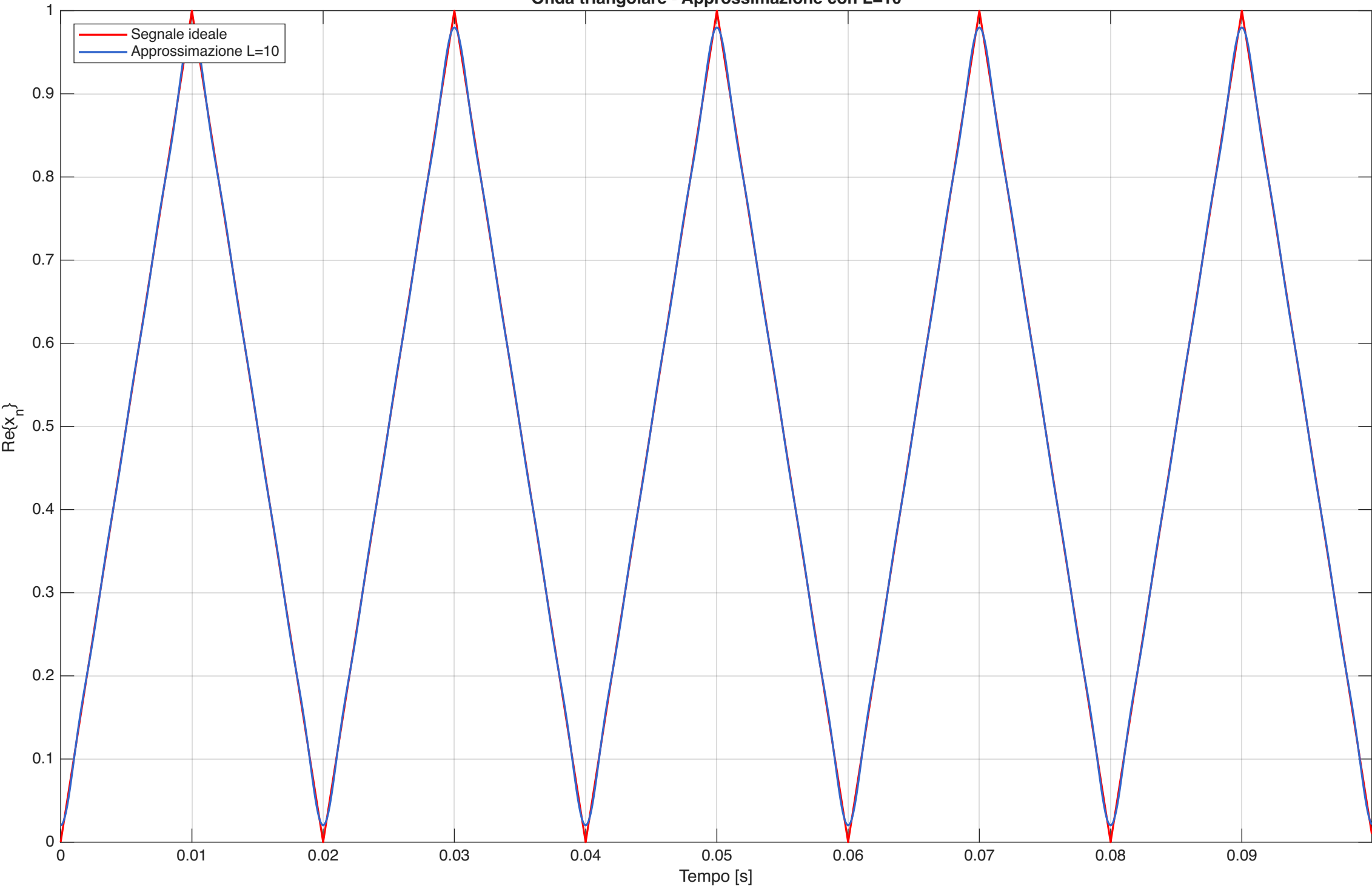
Onda triangolare - Approssimazione con L=10
