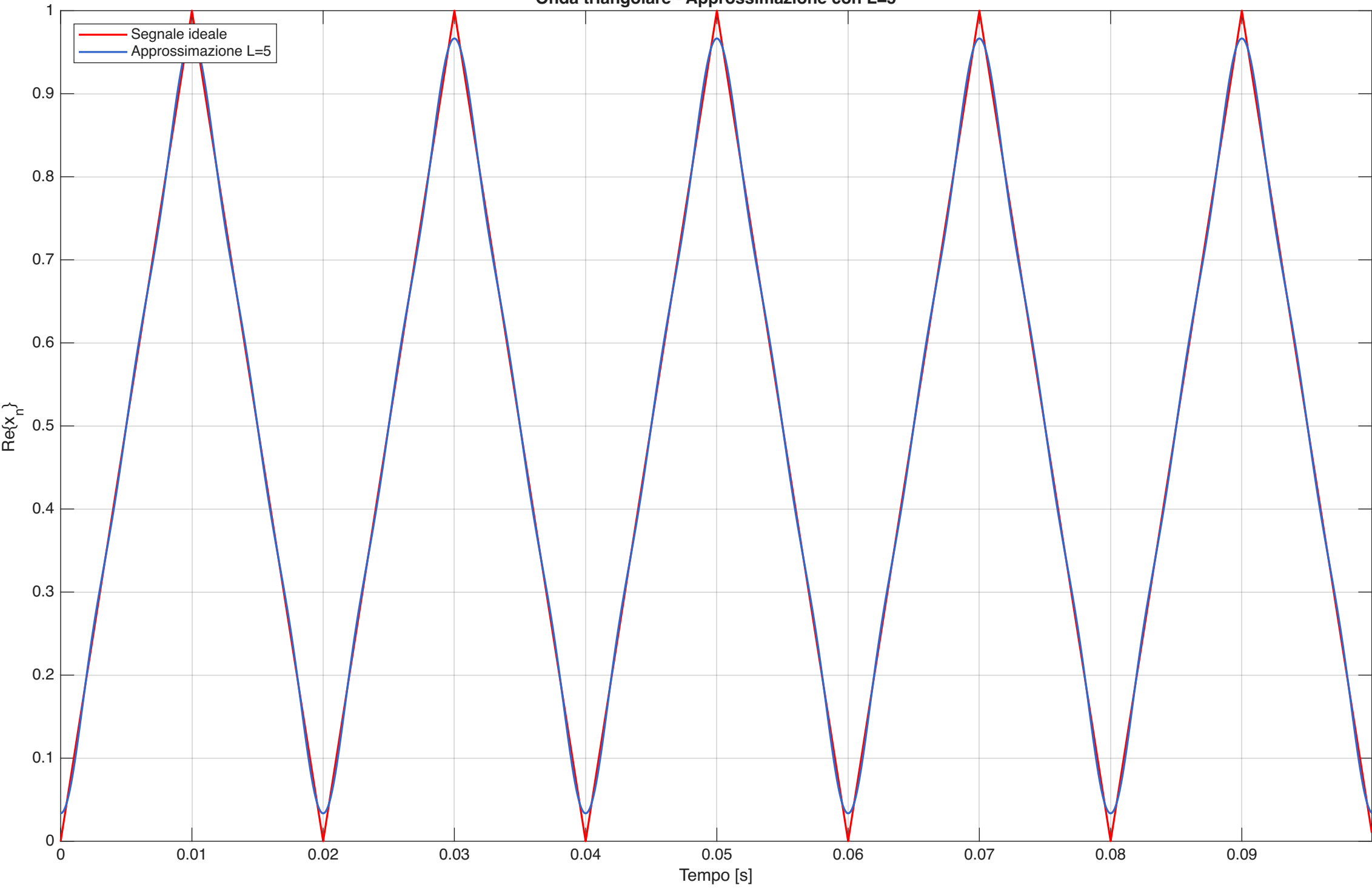
Onda triangolare - Approssimazione con L=5
