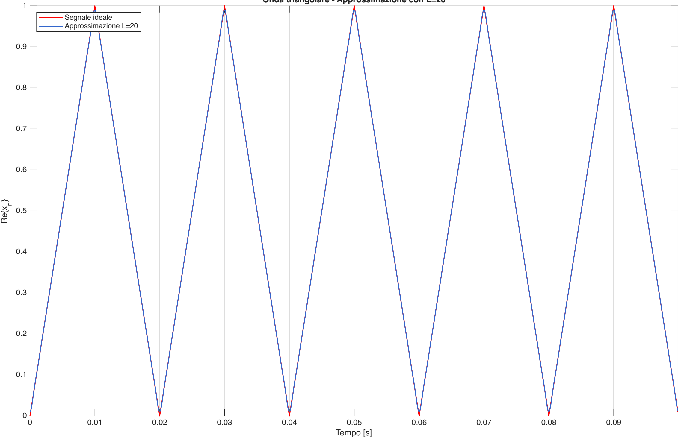
Onda triangolare - Approssimazione con L=20
