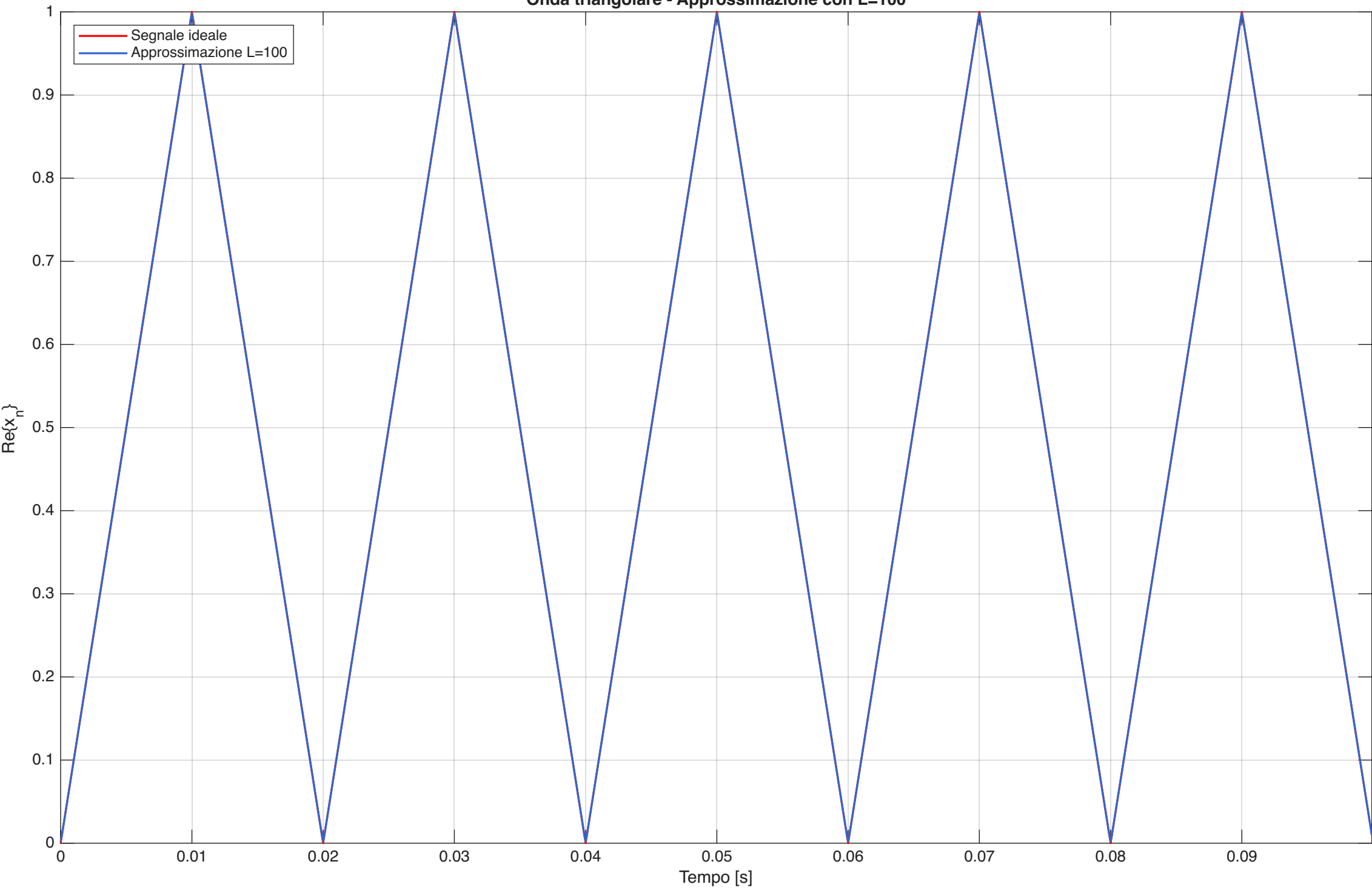
Onda triangolare - Approssimazione con L=100
