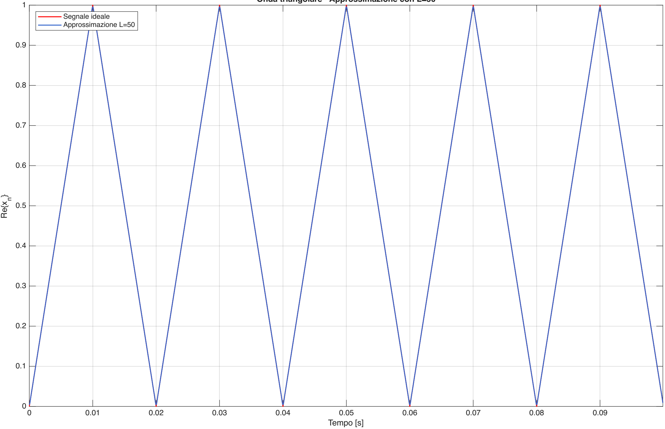
Onda triangolare - Approssimazione con L=50
