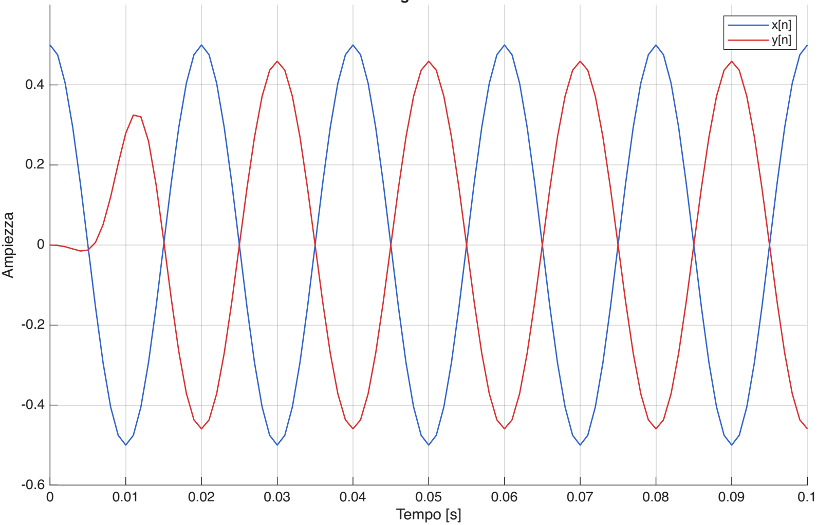
Filtro FIR in virgola fissa — f_0 = 50 Hz
