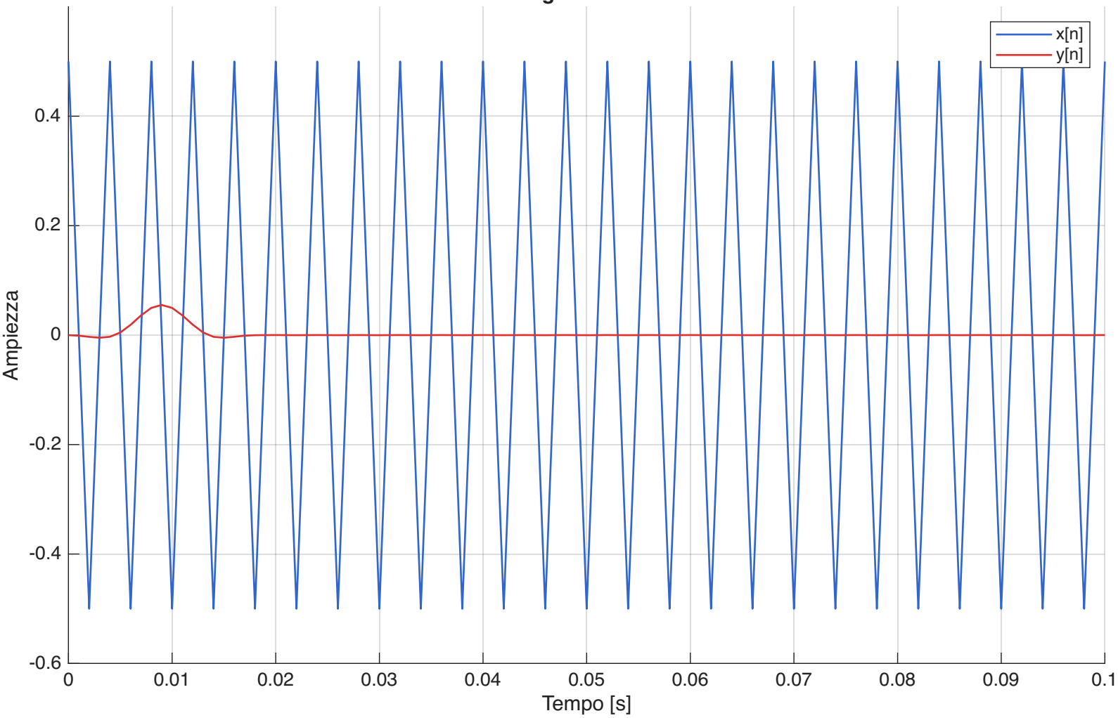
Filtro FIR in virgola fissa — f_0 = 250 Hz
