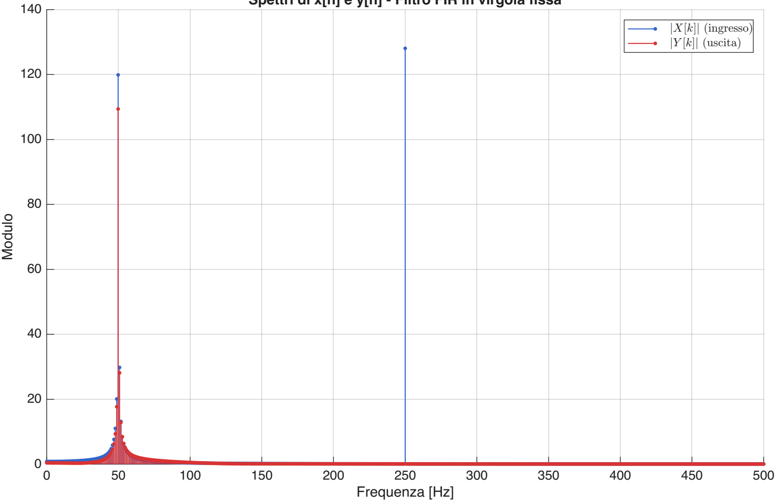
Spettri di x[n] e y[n] - Filtro FIR in virgola fissa
