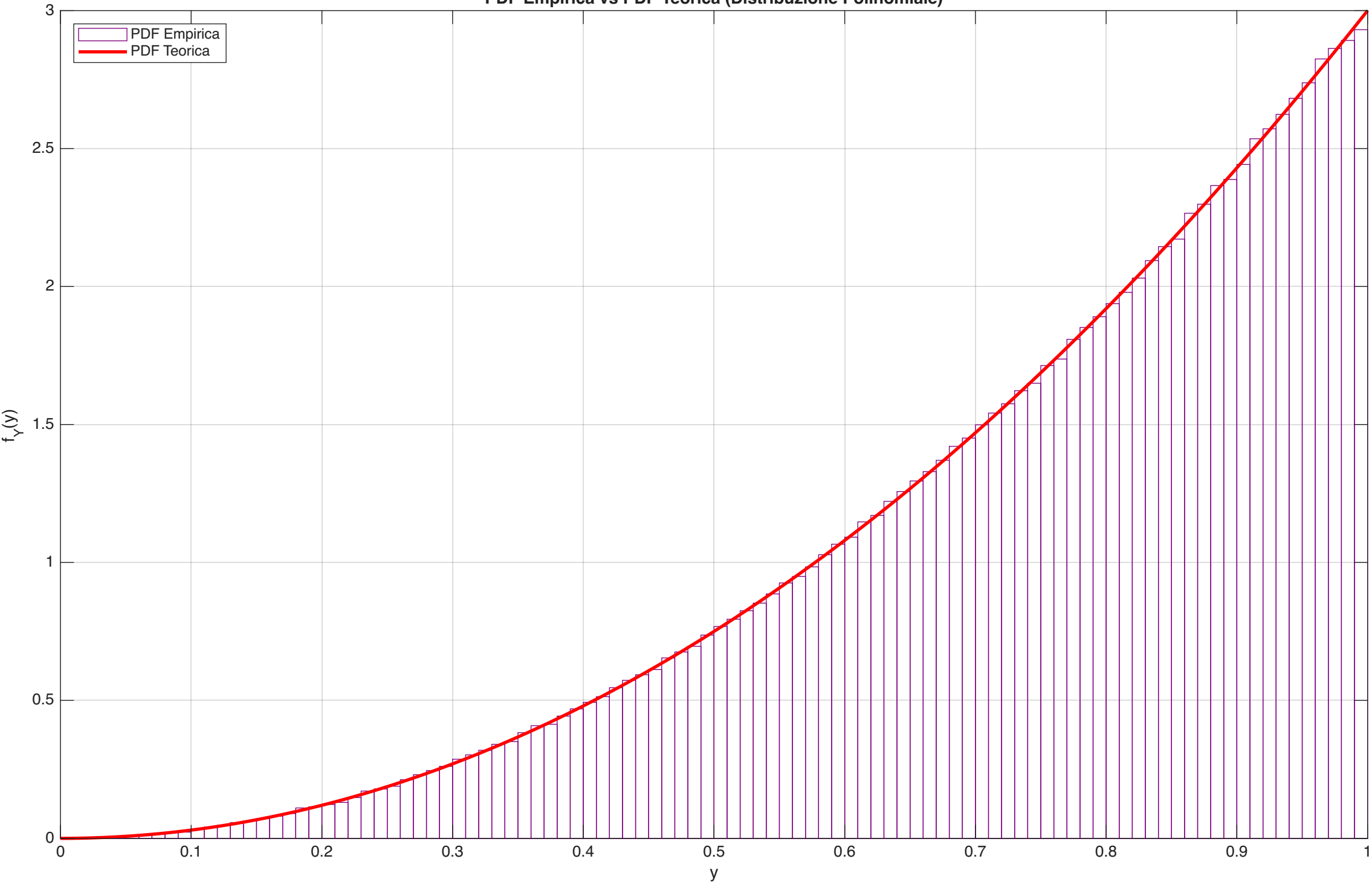
PDF Empirica vs PDF Teorica (Distribuzione Polinomiale)
