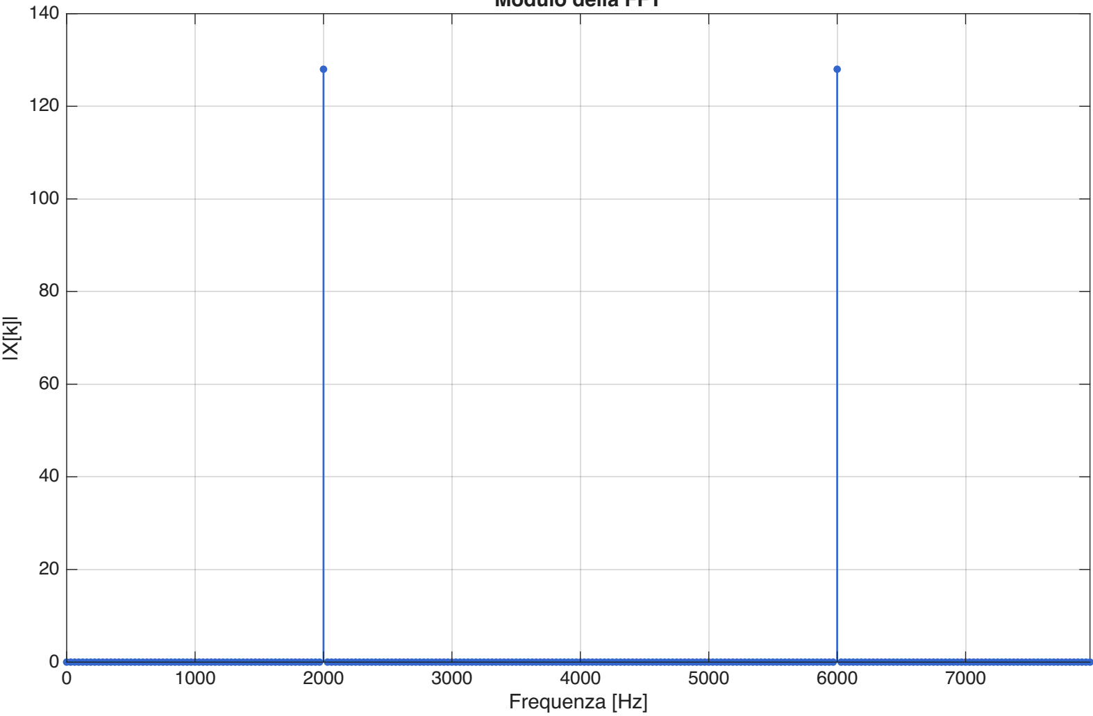
Modulo della FFT
