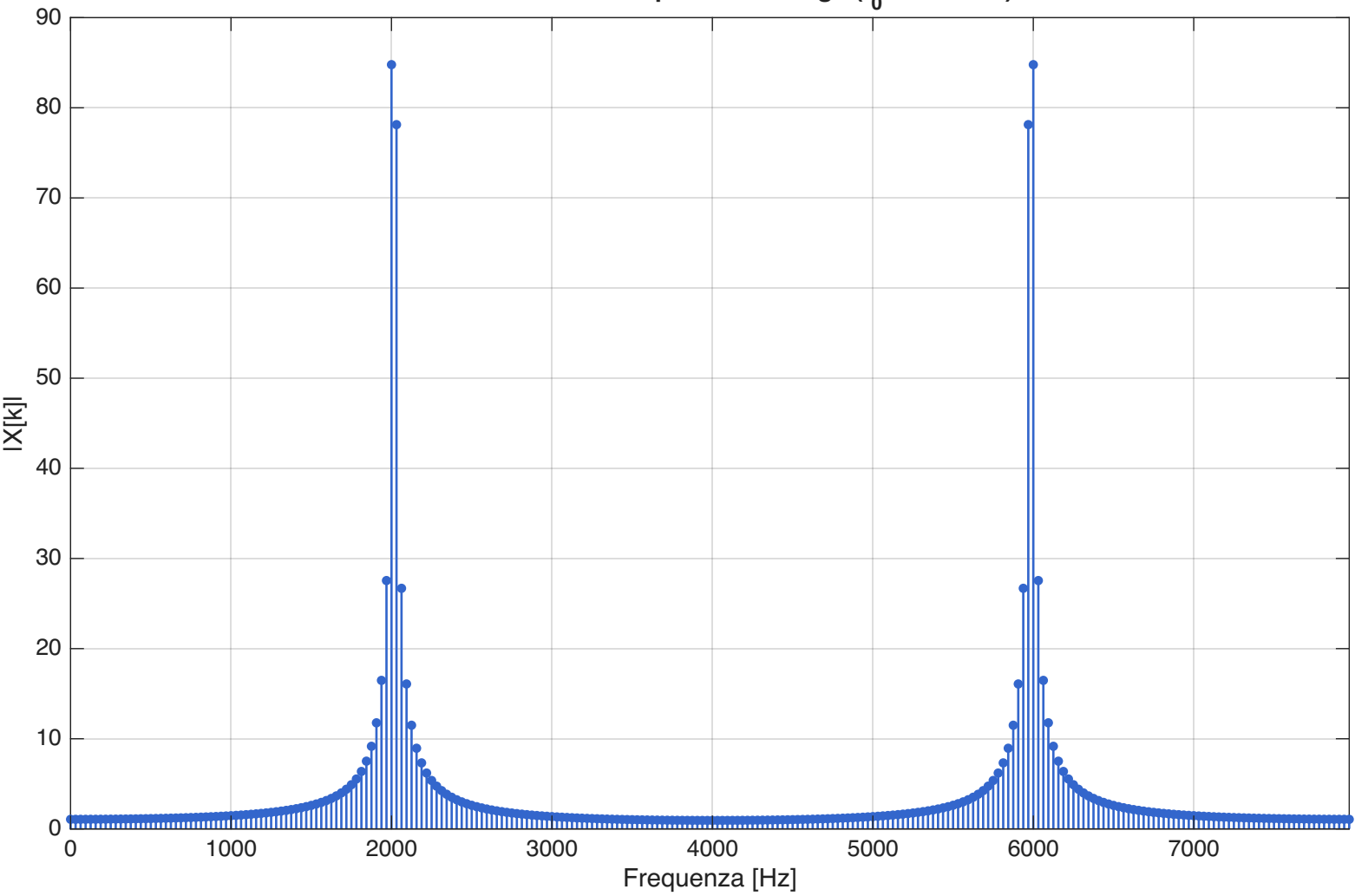
Modulo della FFT - Spectral Leakage ( f_0 = 2015 Hz)
