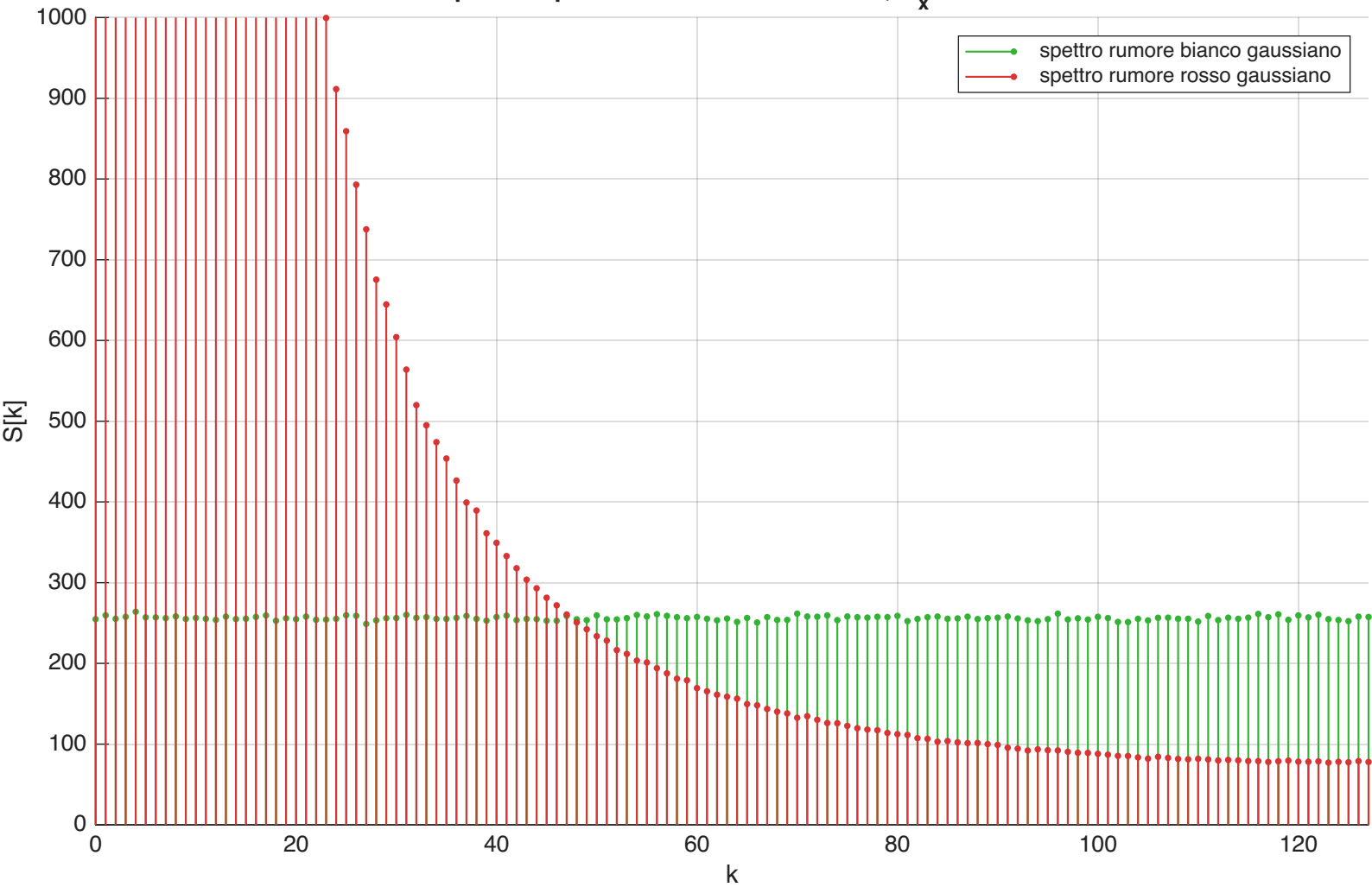
Spettri di potenza medi — Gaussiano, N_x = 10000
