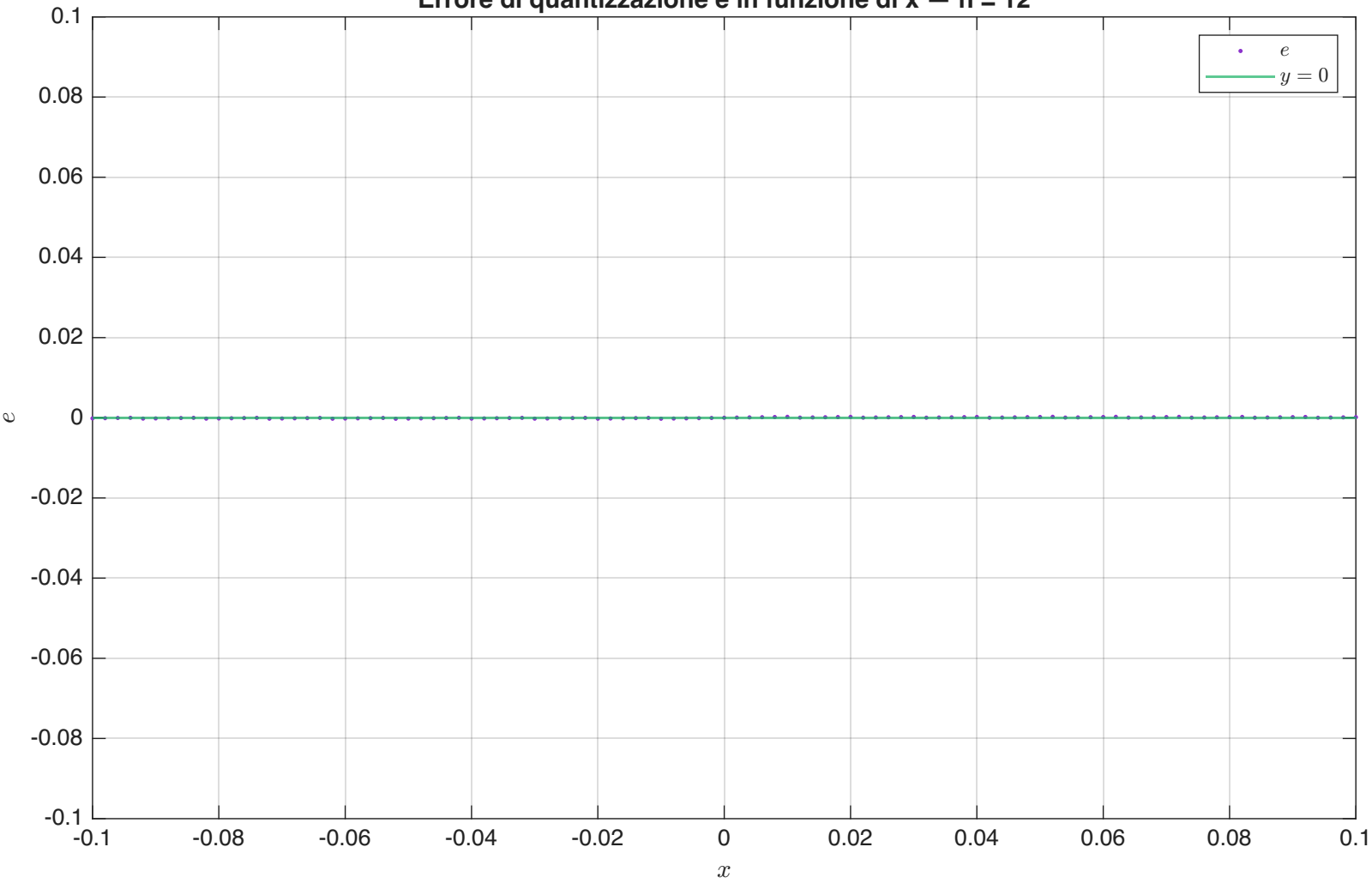
Errore di quantizzazione e in funzione di x — n = 12
