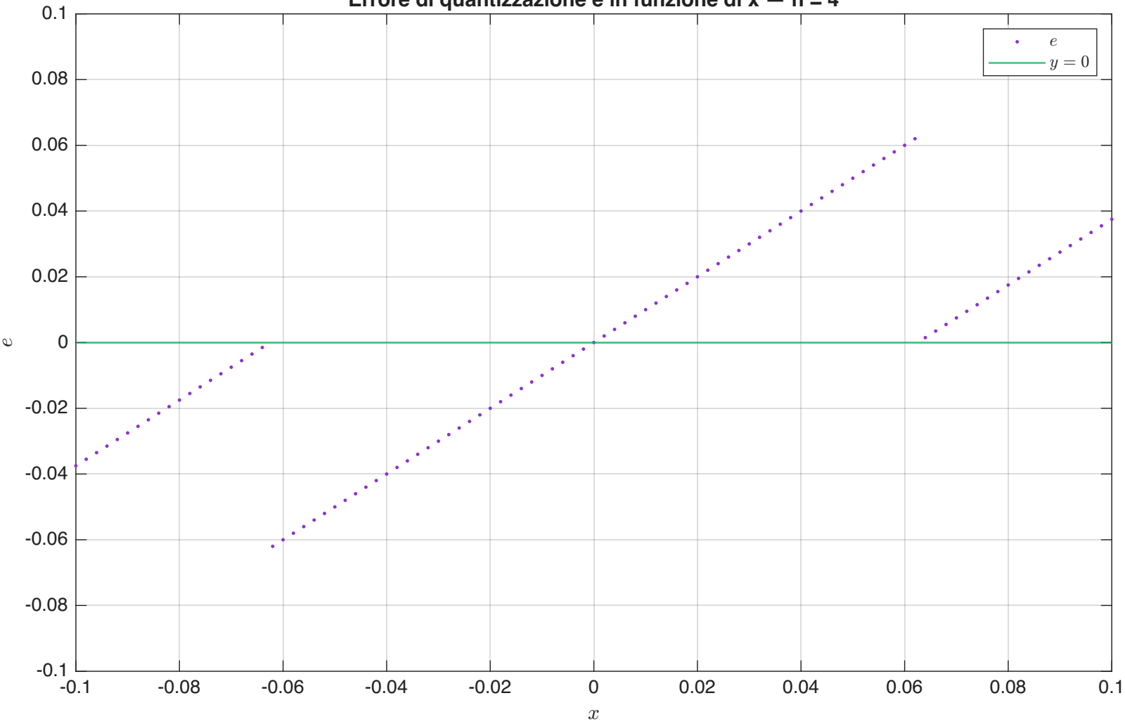
Errore di quantizzazione e in funzione di x — n = 4
