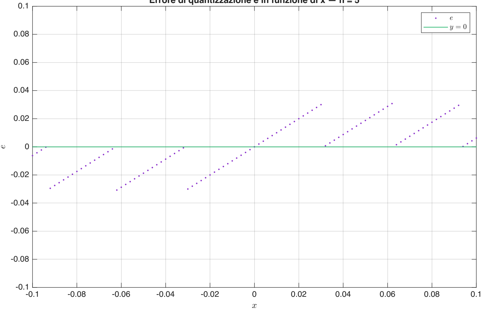
Errore di quantizzazione e in funzione di x — n = 5
