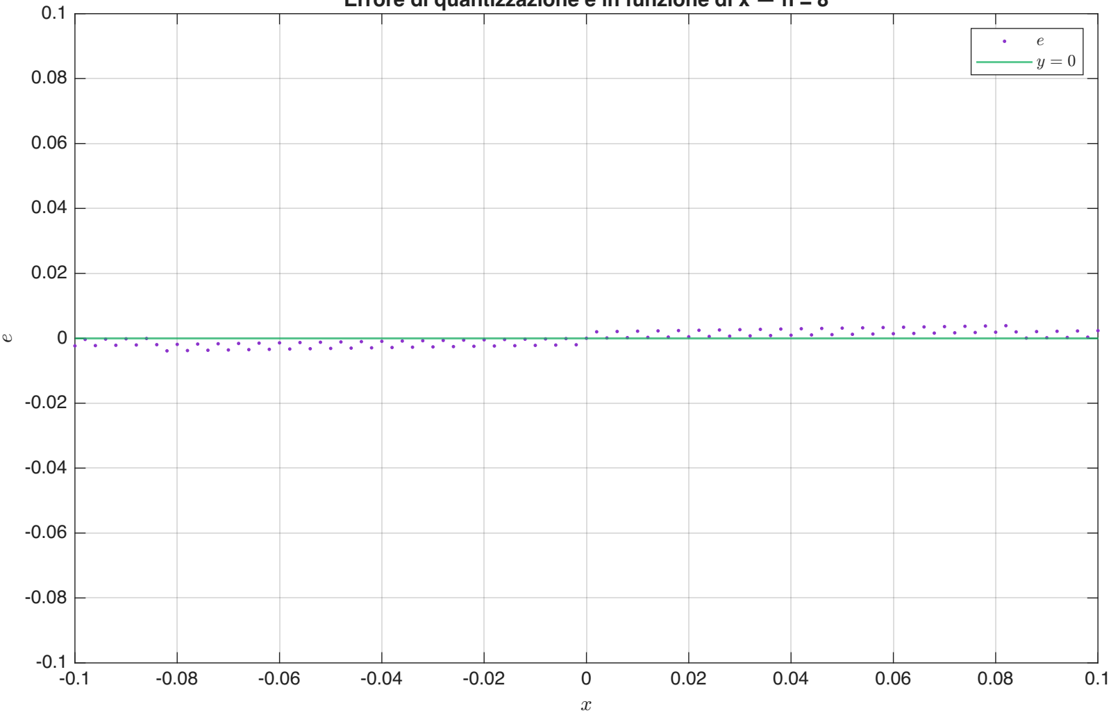
Errore di quantizzazione e in funzione di x — n = 8
