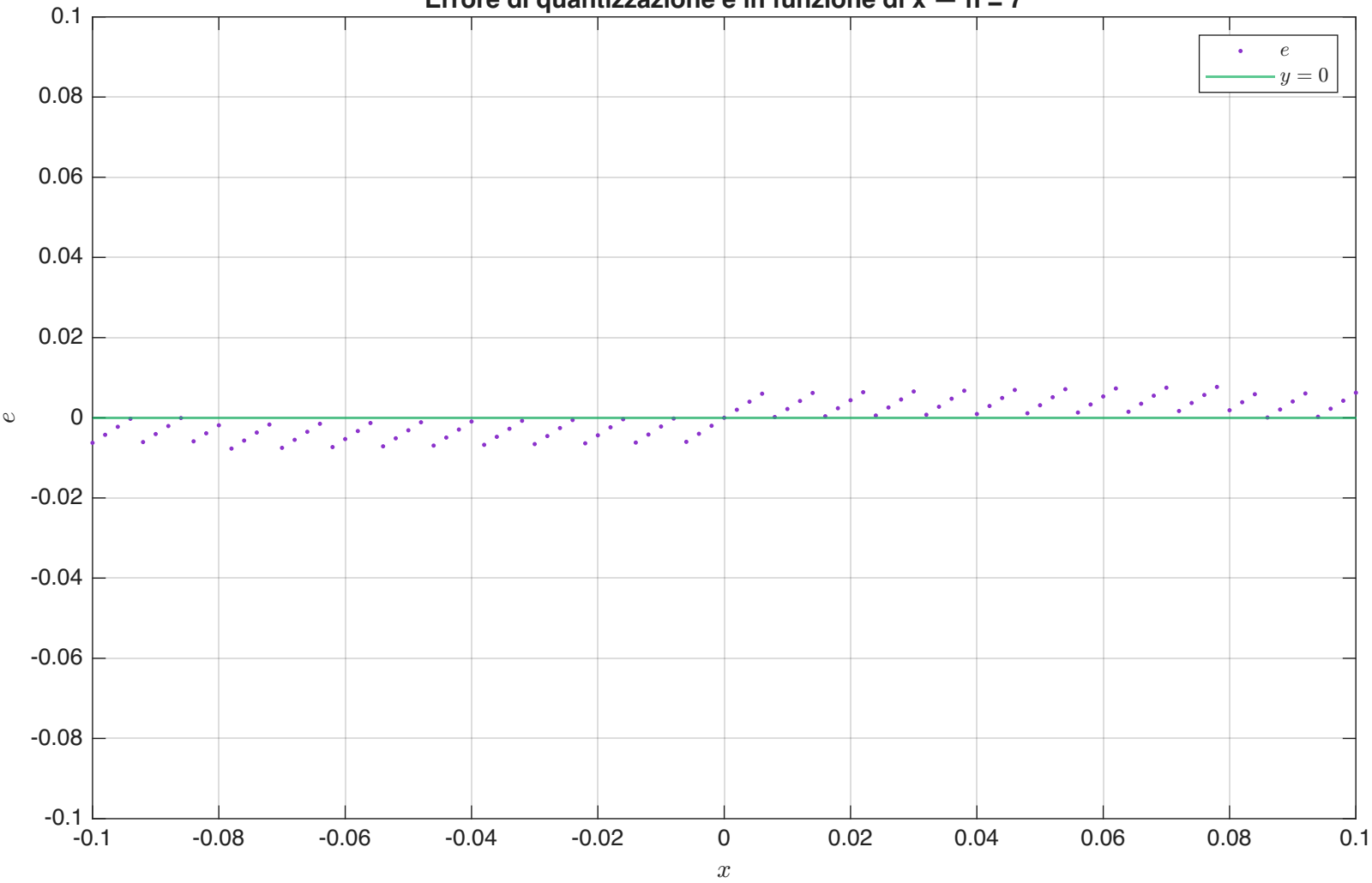
Errore di quantizzazione e in funzione di x — n = 7
