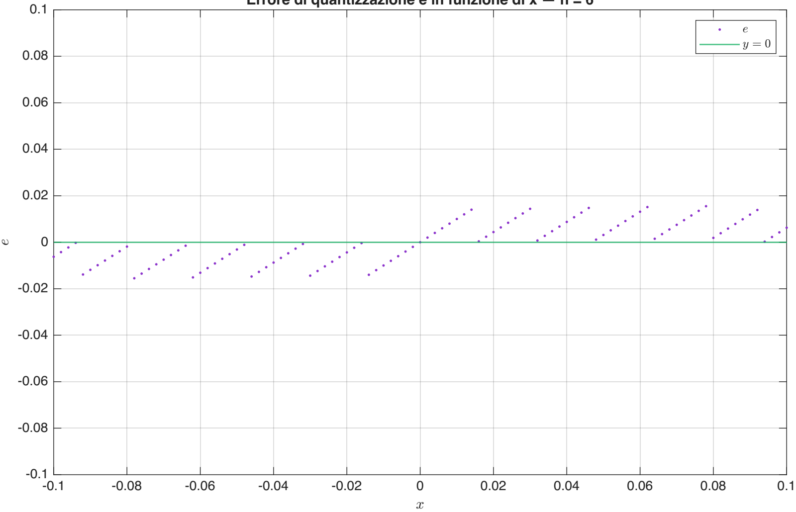
Errore di quantizzazione e in funzione di x — n = 6
