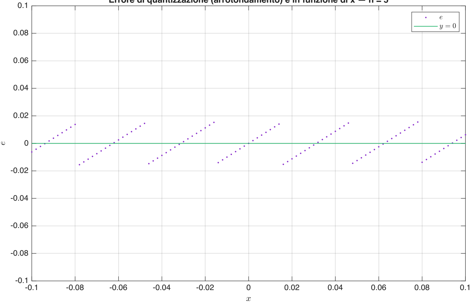
Errore di quantizzazione (arrotondamento) e in funzione di x — n = 5
