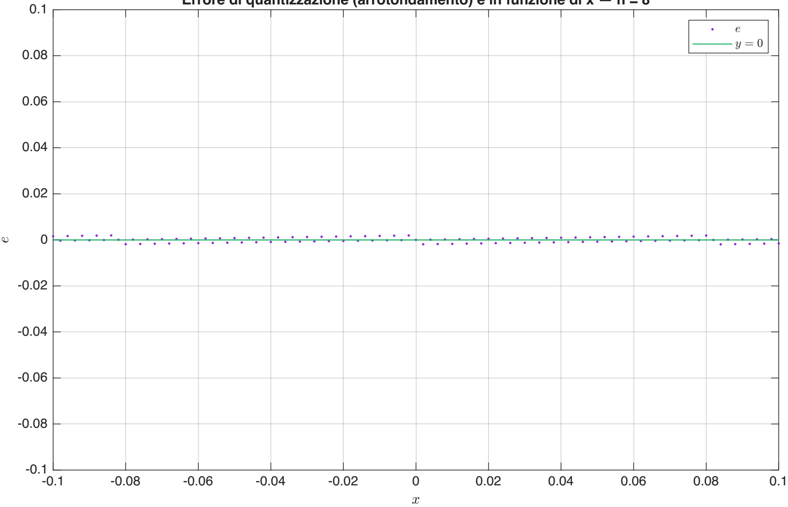
Errore di quantizzazione (arrotondamento) e in funzione di x — n = 8
