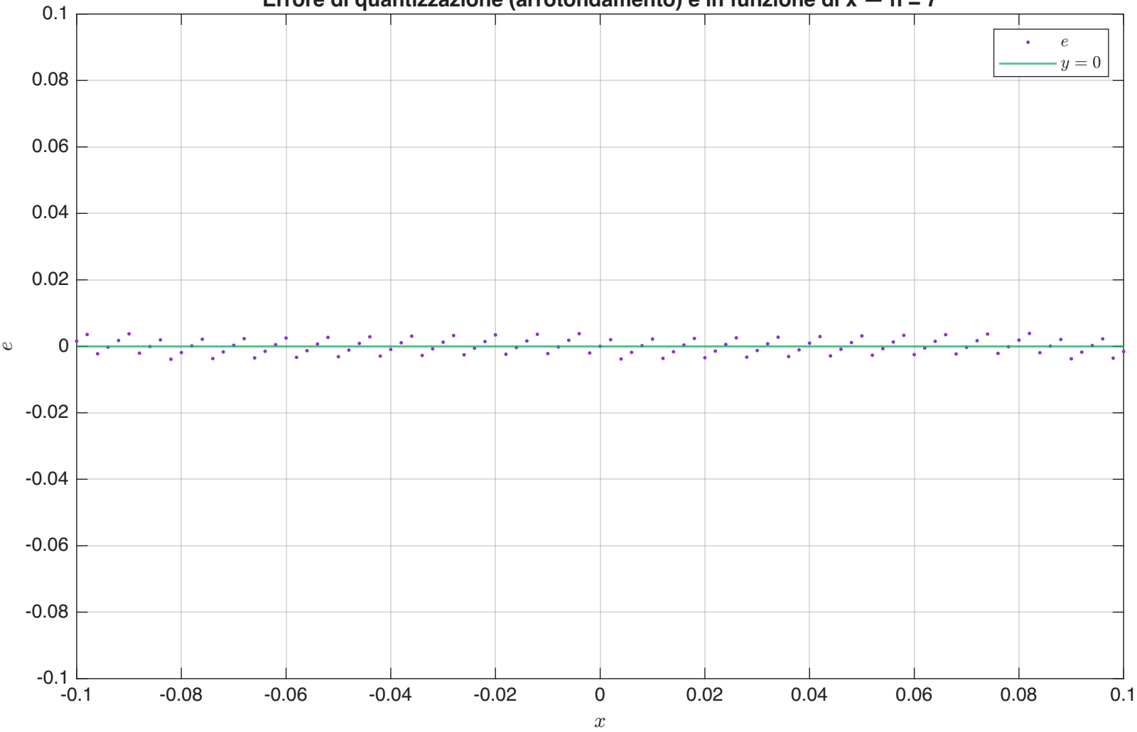
Errore di quantizzazione (arrotondamento) e in funzione di x — n = 7
