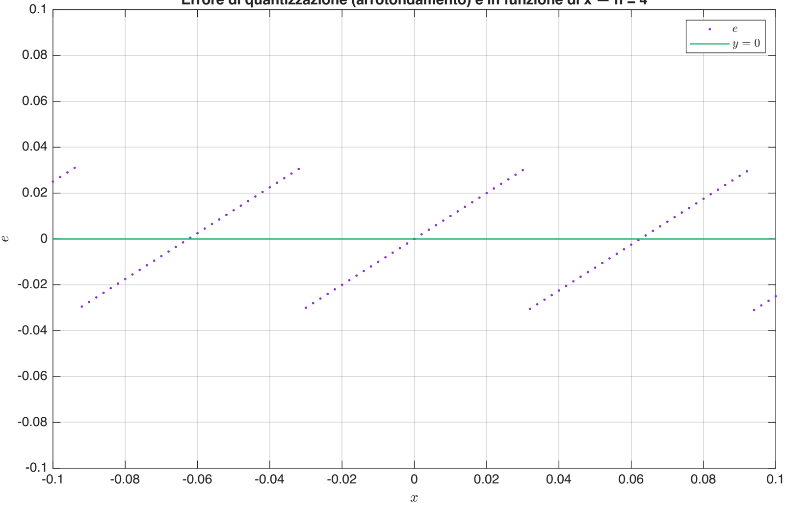
Errore di quantizzazione (arrotondamento) e in funzione di x — n = 4
