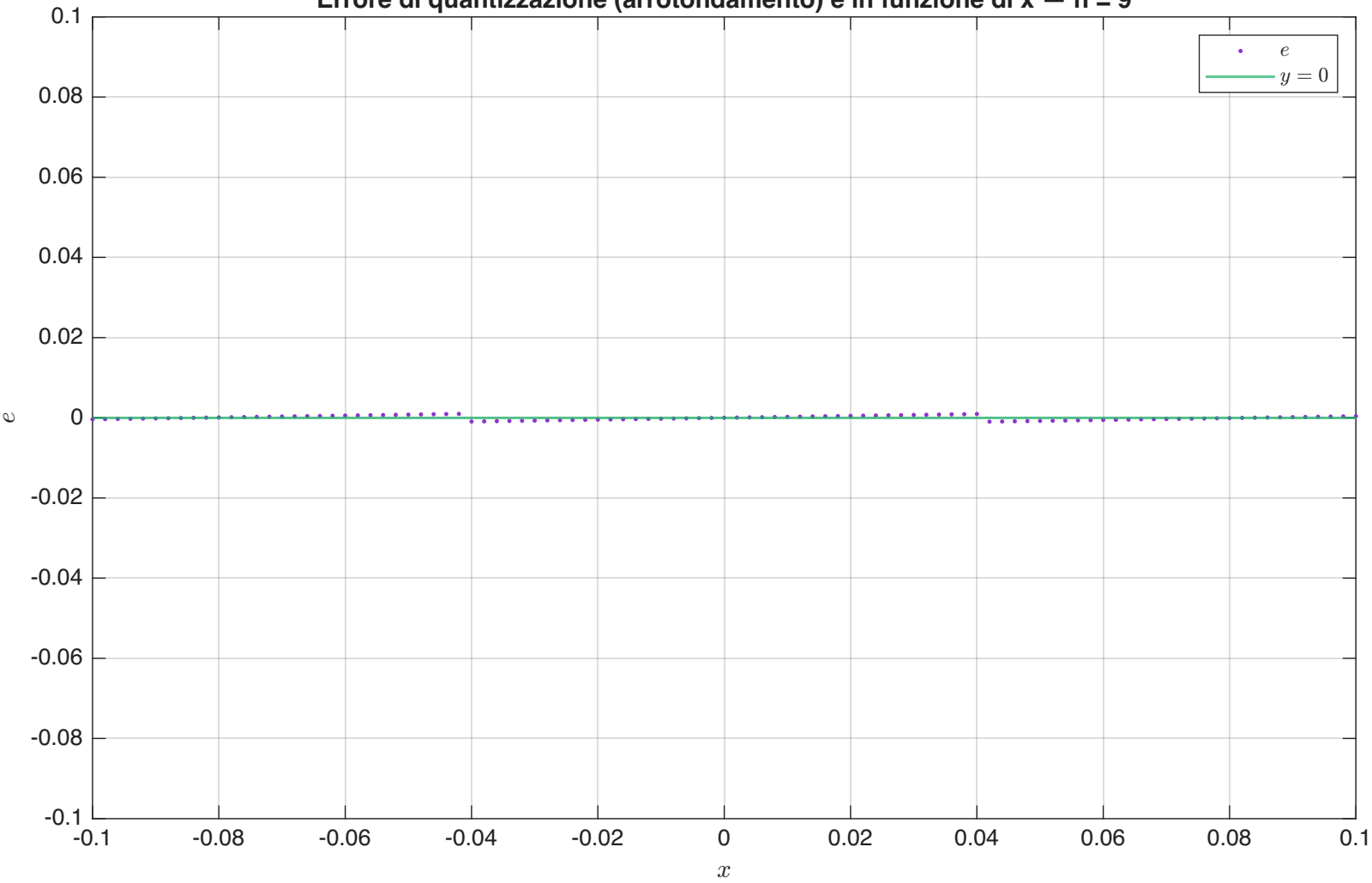
Errore di quantizzazione (arrotondamento) e in funzione di x — n = 9
