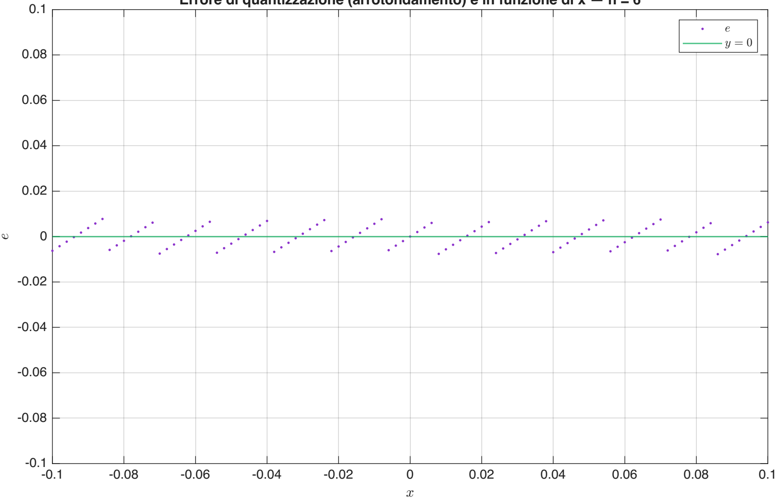
Errore di quantizzazione (arrotondamento) e in funzione di x — n = 6
