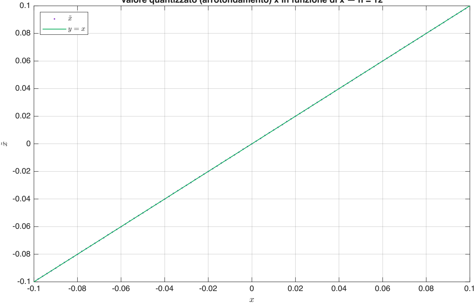
Valore quantizzato (arrotondamento) \tilde{x} in funzione di x — n = 12
