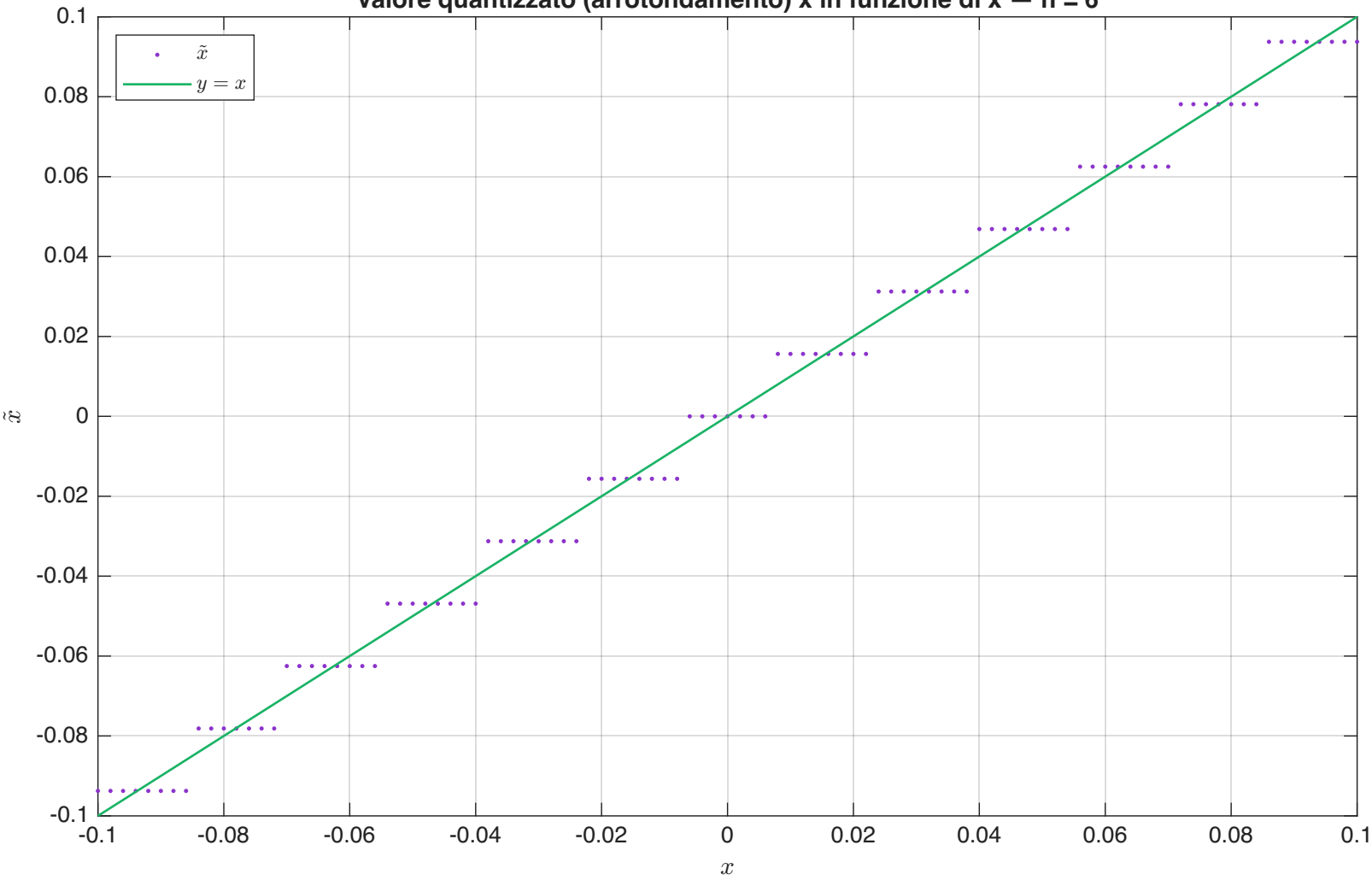
Valore quantizzato (arrotondamento) \hat{x} in funzione di x — n = 6
