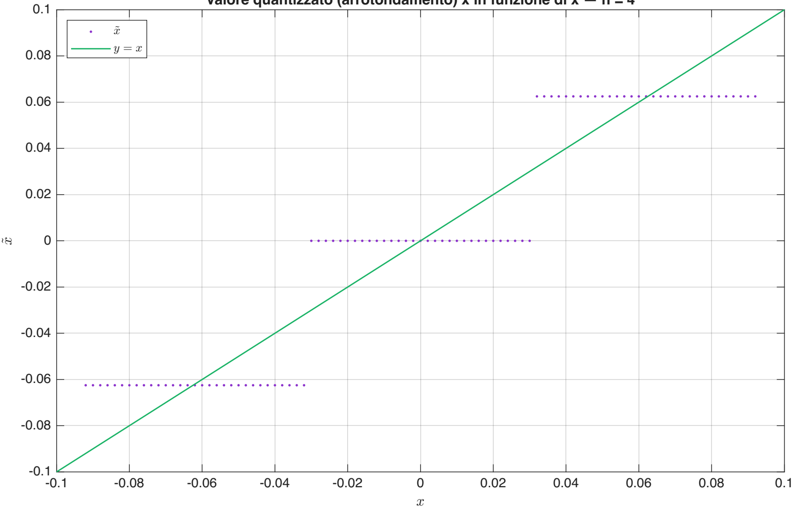
Valore quantizzato (arrotondamento) \hat{x} in funzione di x — n = 4
