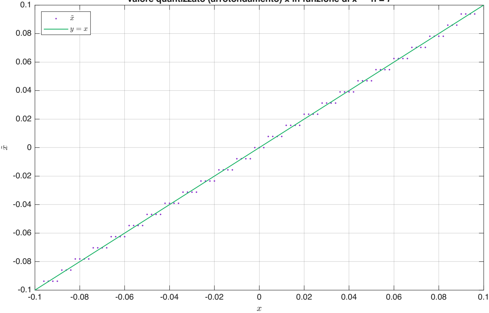
Valore quantizzato (arrotondamento) \hat{x} in funzione di x — n = 7
