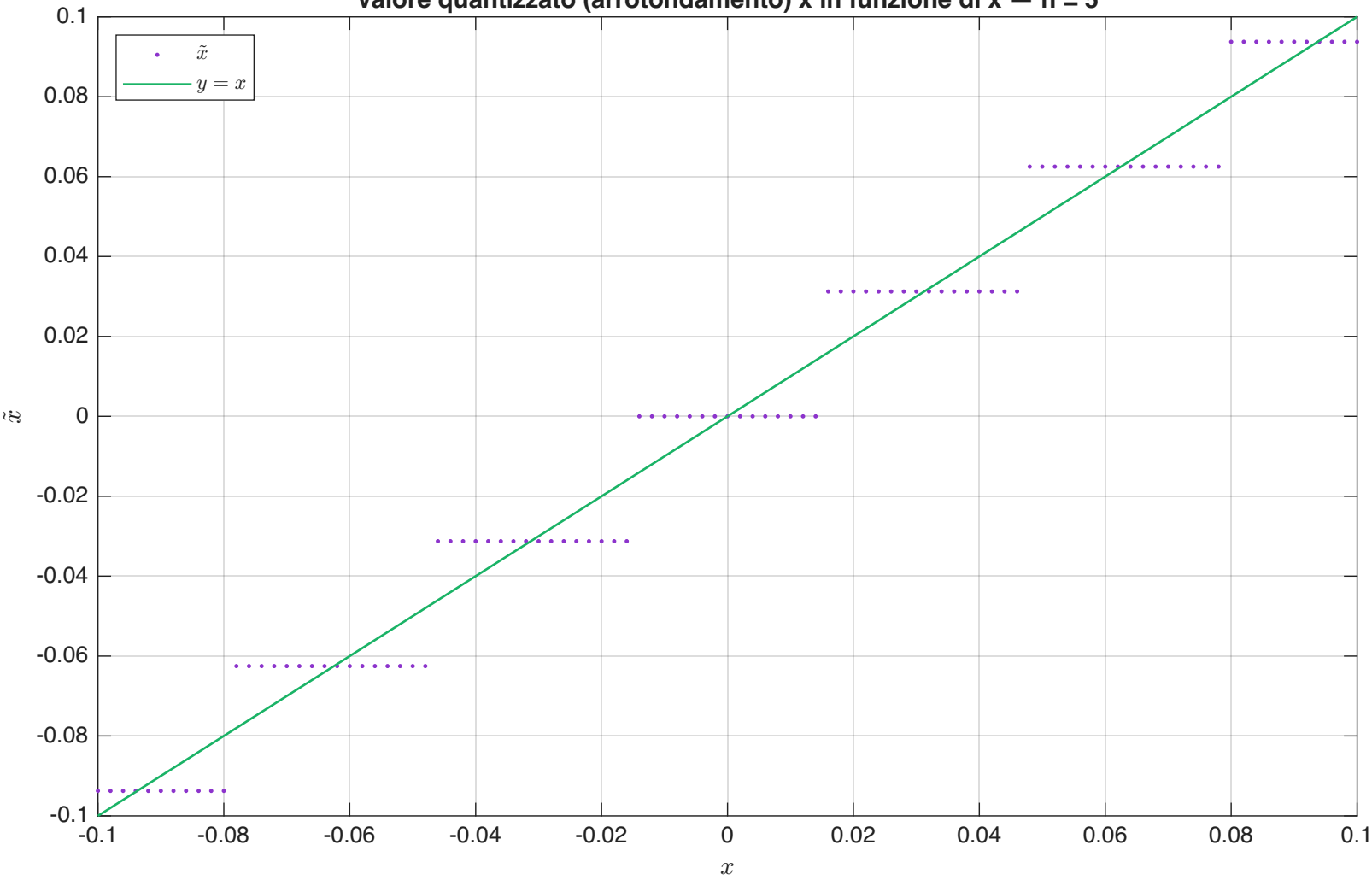
Valore quantizzato (arrotondamento) \hat{x} in funzione di x — n = 5
