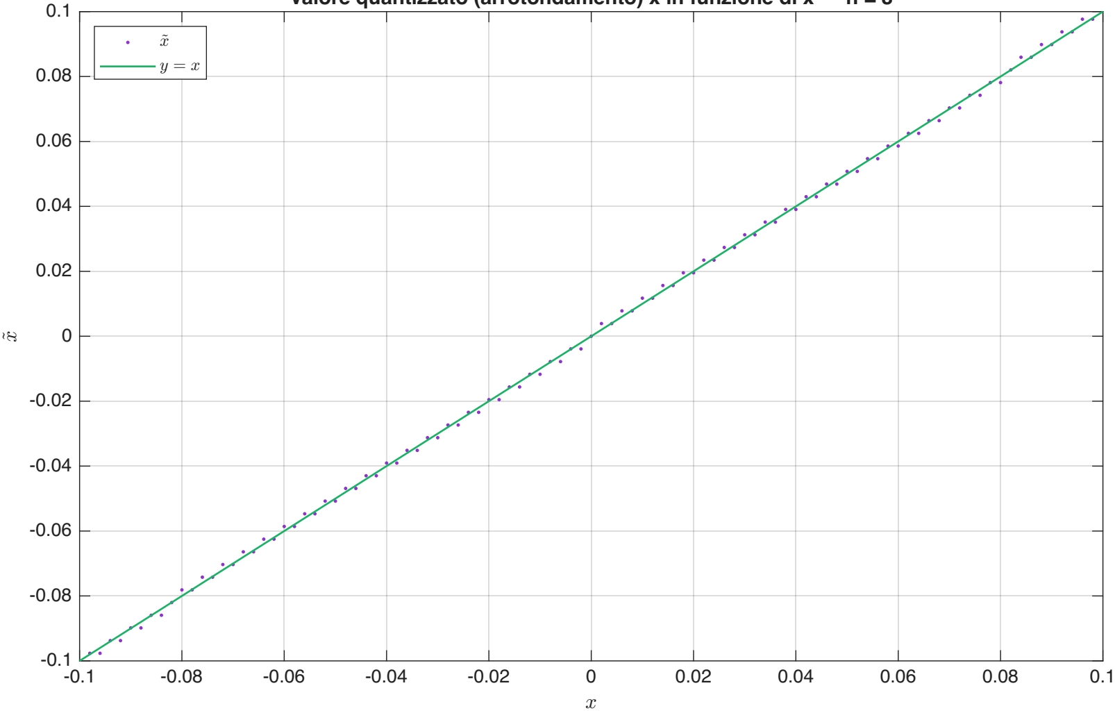
Valore quantizzato (arrotondamento) \hat{x} in funzione di x — n = 8
