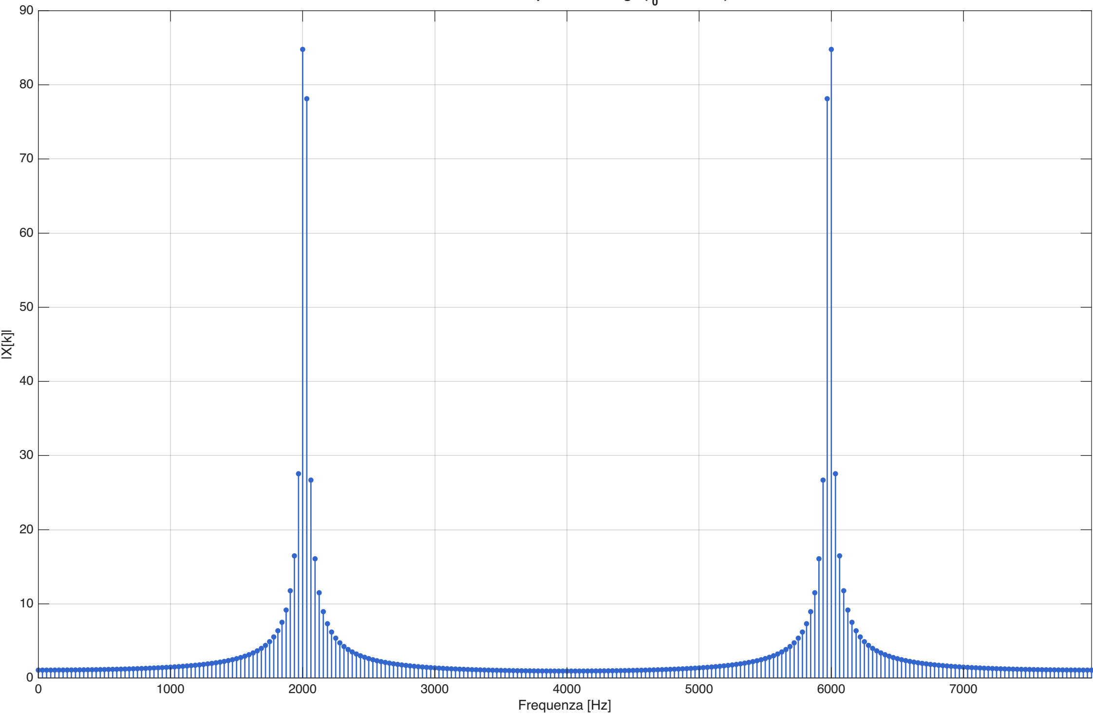
Modulo della DFT - Spectral Leakage ( f_0 = 2015 Hz)
