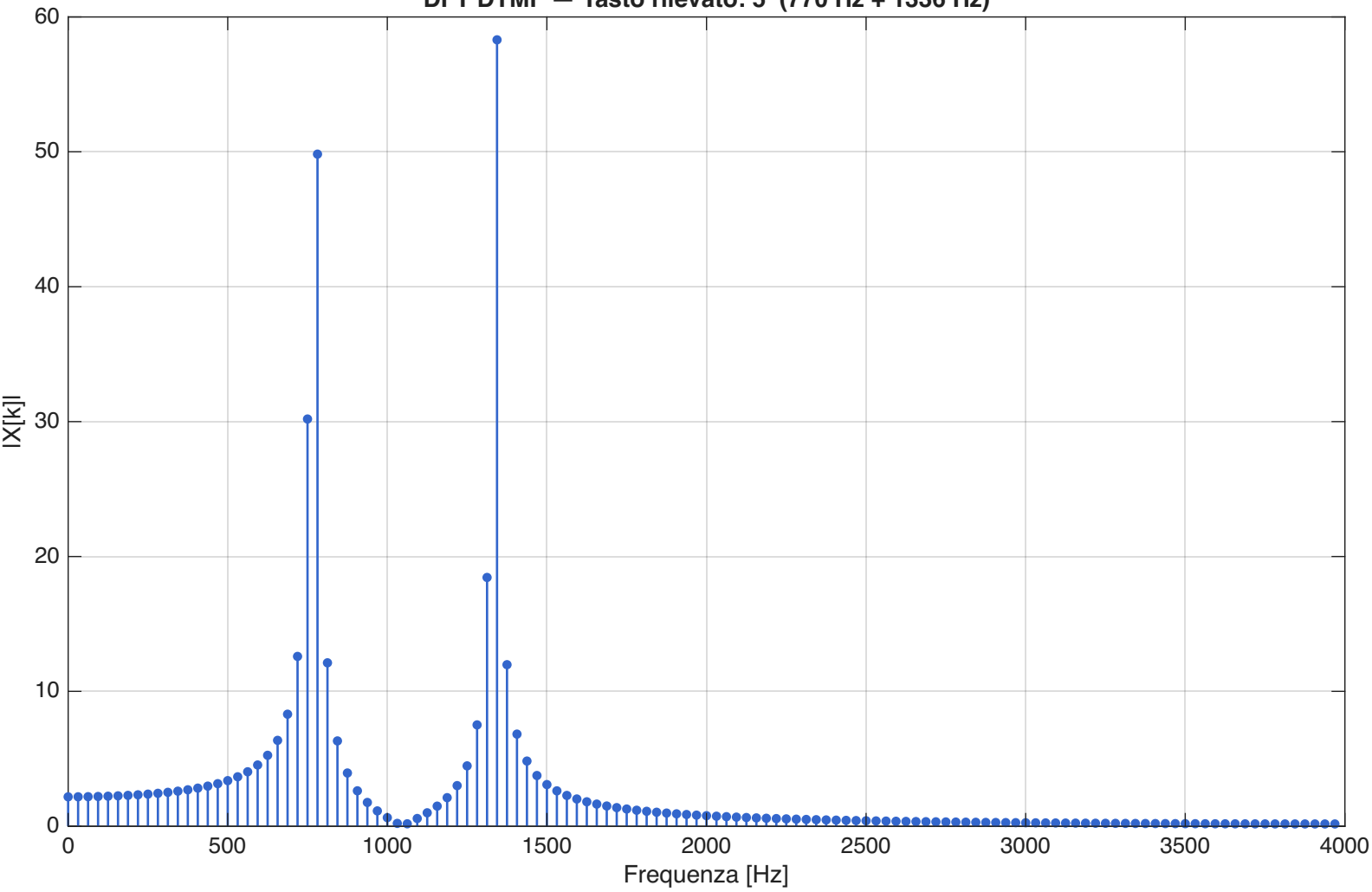
DFT DTMF — Tasto rilevato: 5 (770 Hz + 1336 Hz)
