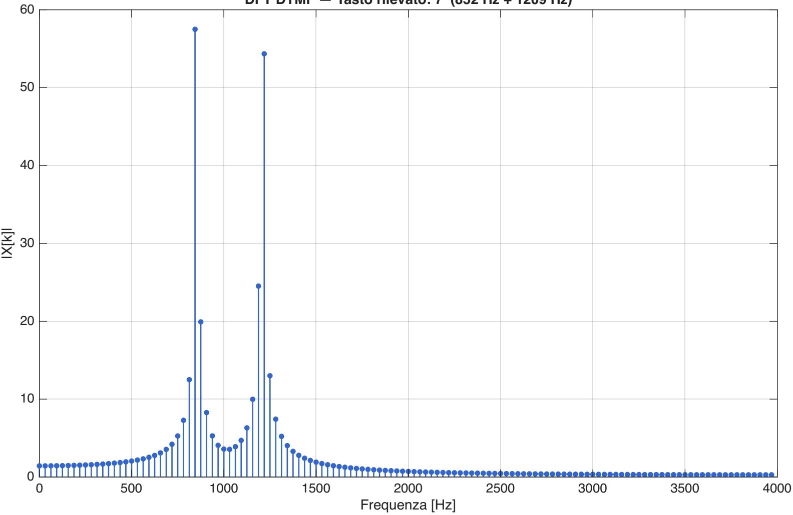
DFT DTMF — Tasto rilevato: 7 (852 Hz + 1209 Hz)
