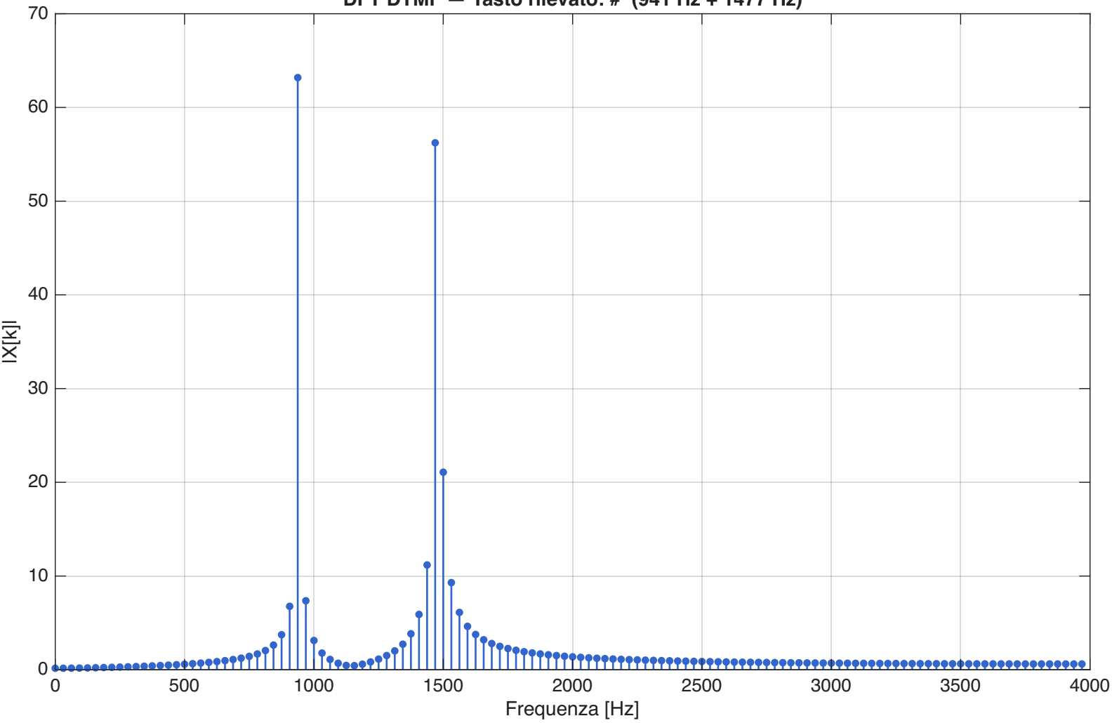
DFT DTMF — Tasto rilevato: # (941 Hz + 1477 Hz)
