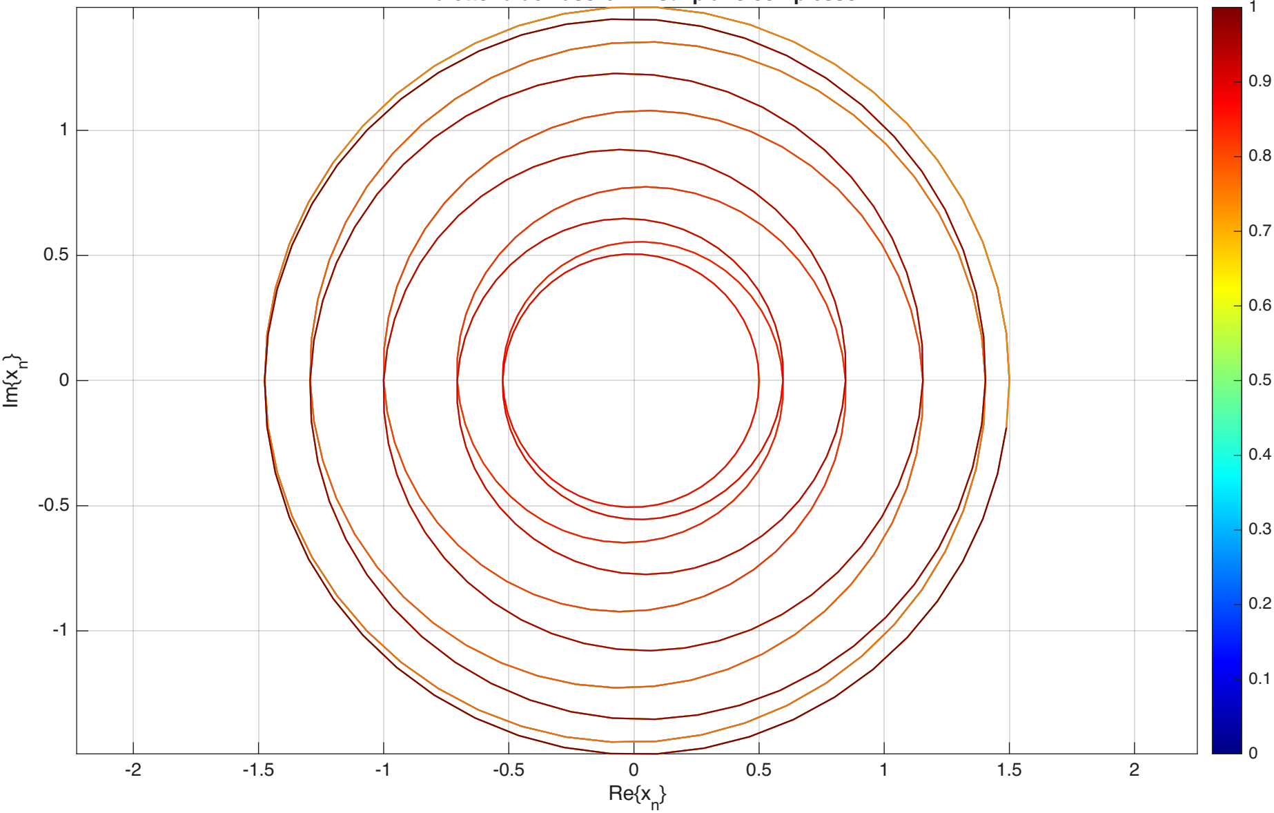
Traiettoria del fasore AM sul piano complesso
