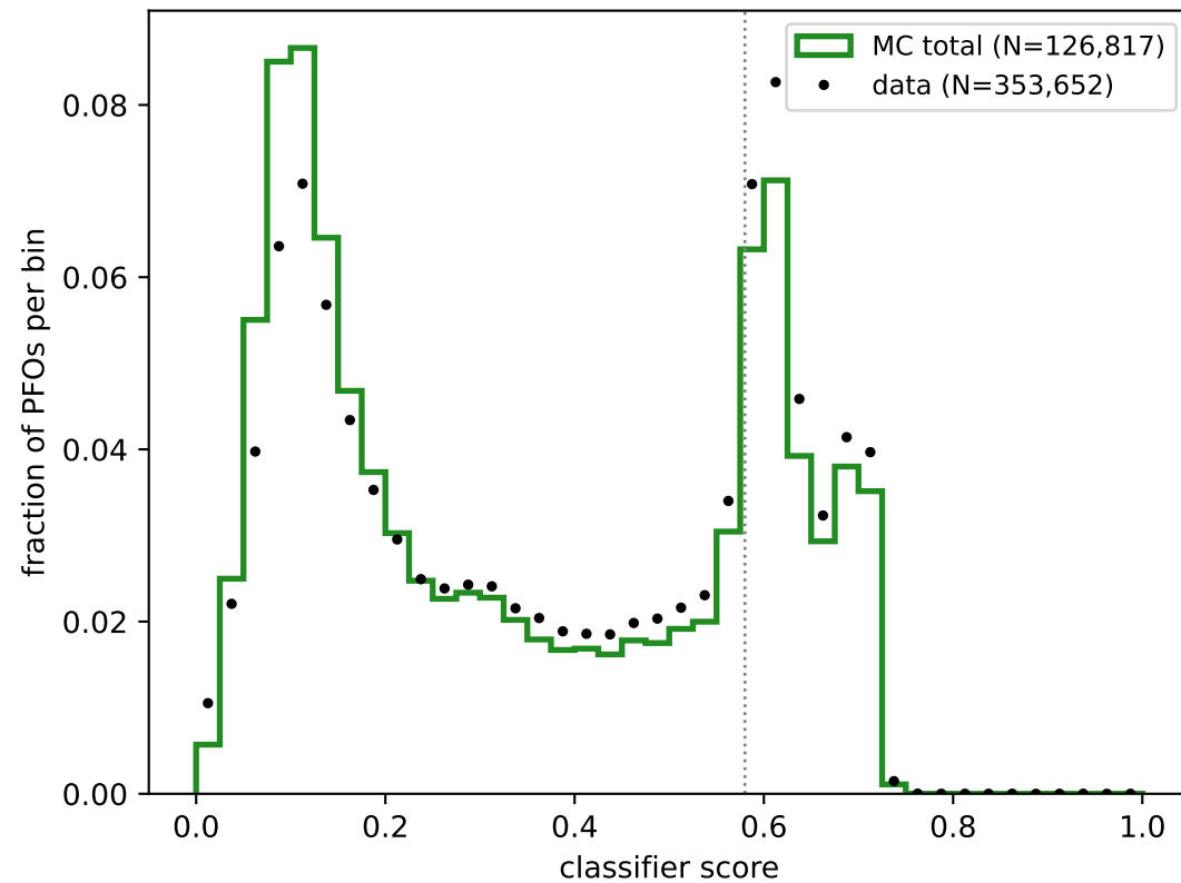
MLP
