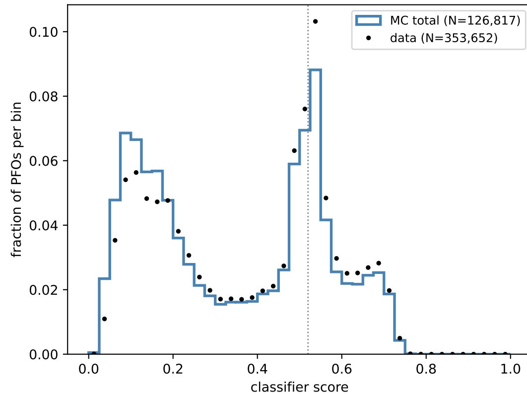
CNN
