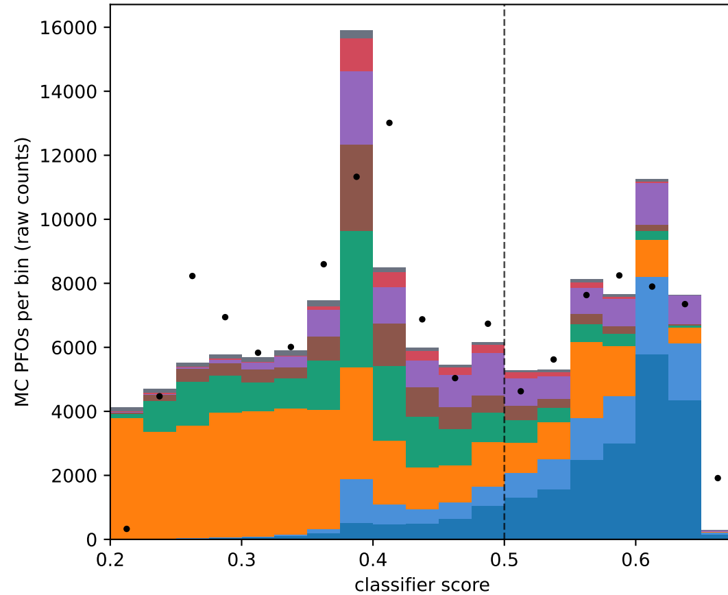
MLP
