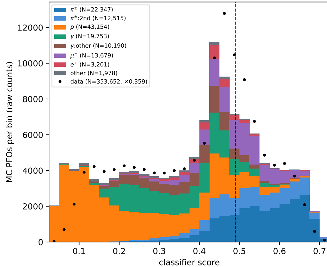
CNN
