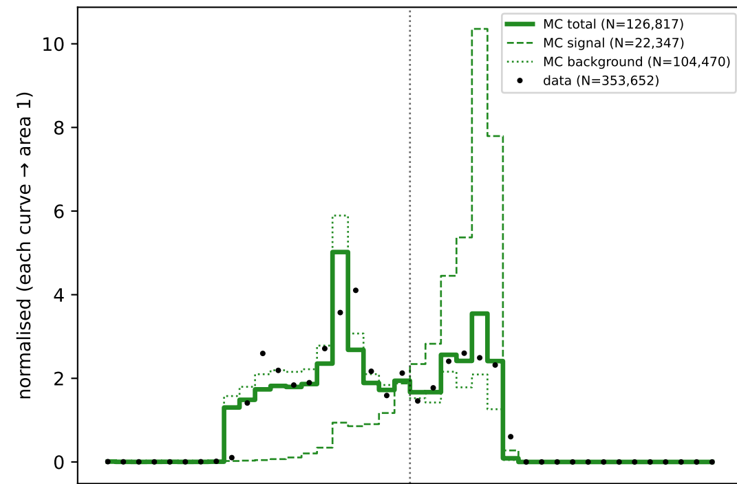
MLP
