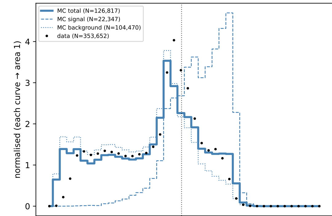
CNN
