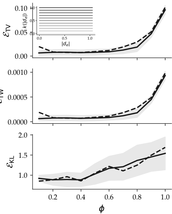
DeGroot
