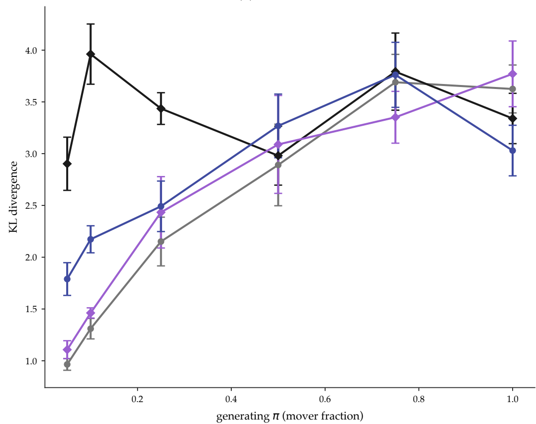
(d) time-series KLD
