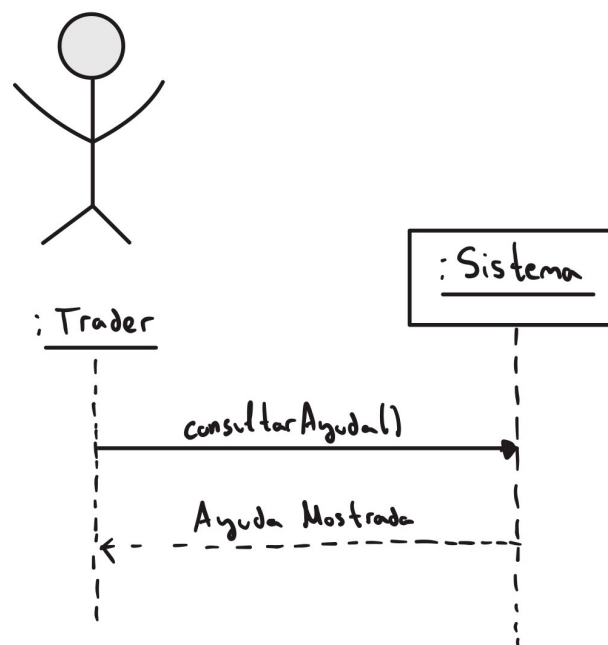
Figura 19: Diagrama de secuencia del sistema para el CU18.
