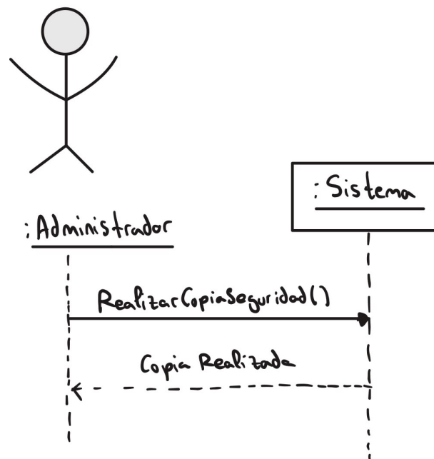
Figura 20: Diagrama de secuencia del sistema para el CU19.
