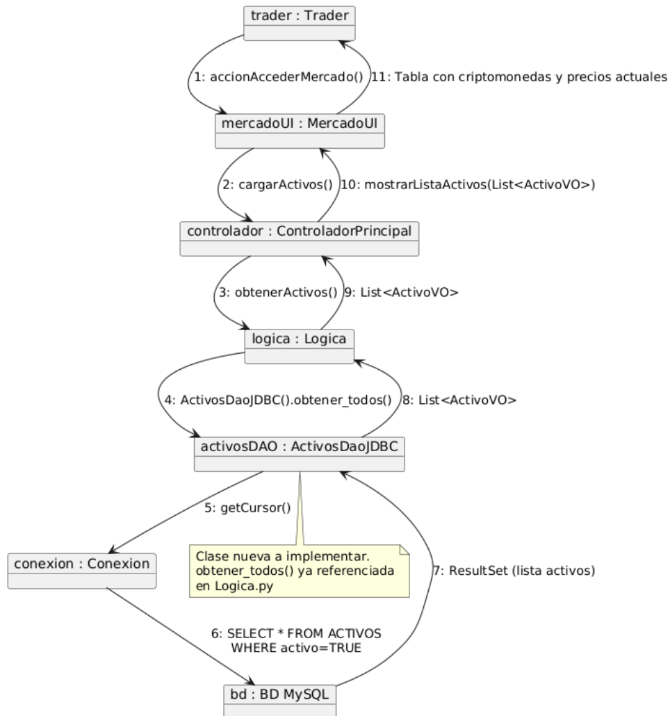
CU4: Consultar criptomonedas (Diagrama de Colaboración)
