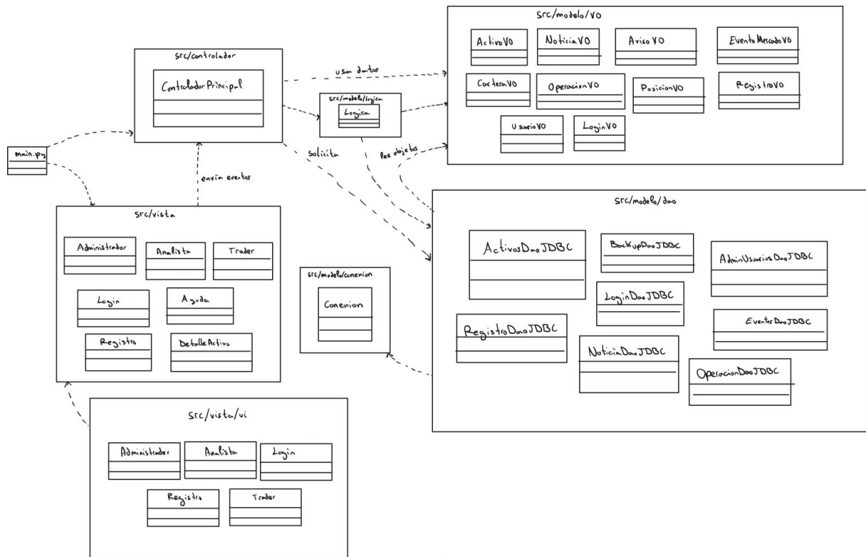
Figura 14: Diagrama de paquetes
