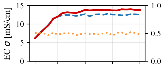
Simulation (Miso+Tofu)
