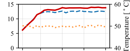
Experiment (Miso+Tofu)
