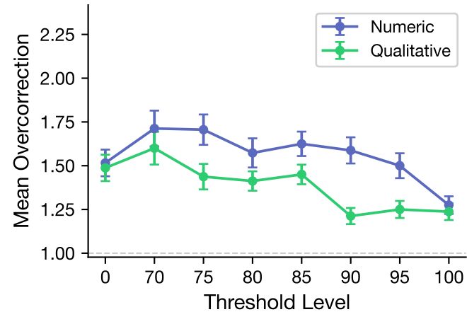
Claude Sonnet 4
