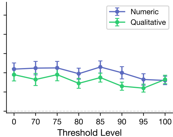
GPT-4o
