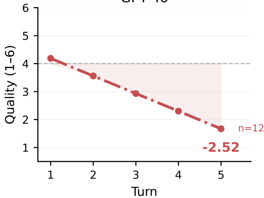
GPT-4o
