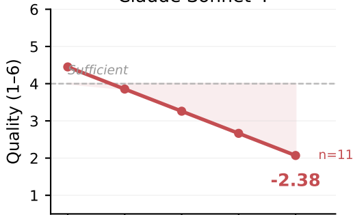
Claude Sonnet 4
