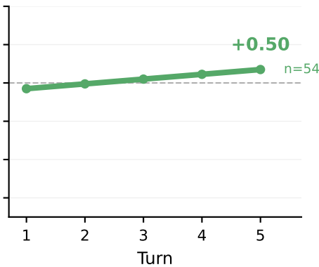
Llama 3.3 70B
