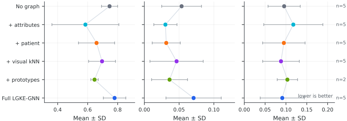
pAUC
