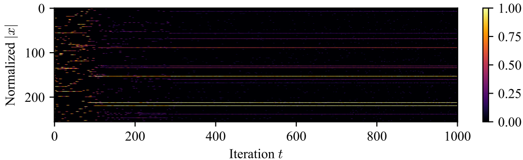
IHT
