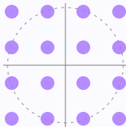
16-QAM
