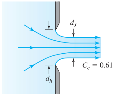
圖 15. 無內壁延伸的開口 [3, p.521]
