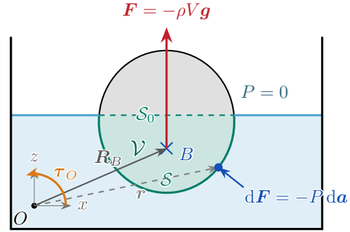
圖 2. 浮力作用線與沉水體積的幾何中心。
