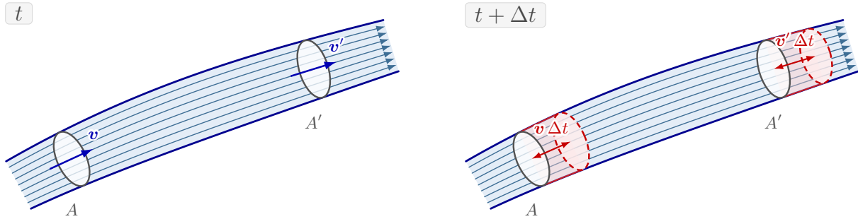
圖 6. 流體在時刻 t 與 t + \Delta t 之間的動量變化。
