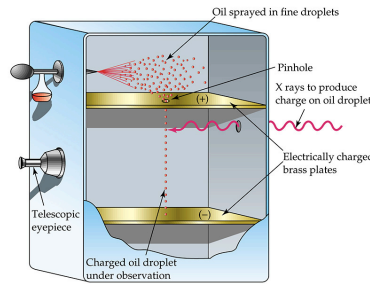
圖 23. 密立坎油滴實驗示意圖 30
