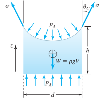
圖 9. 表面張力在兩垂直板之間的作用力圖。[3, p.91]
