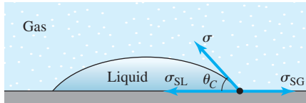
圖 7. 液面示意圖。上圖 \theta_c 即為 \theta 。[3, p. 90]
