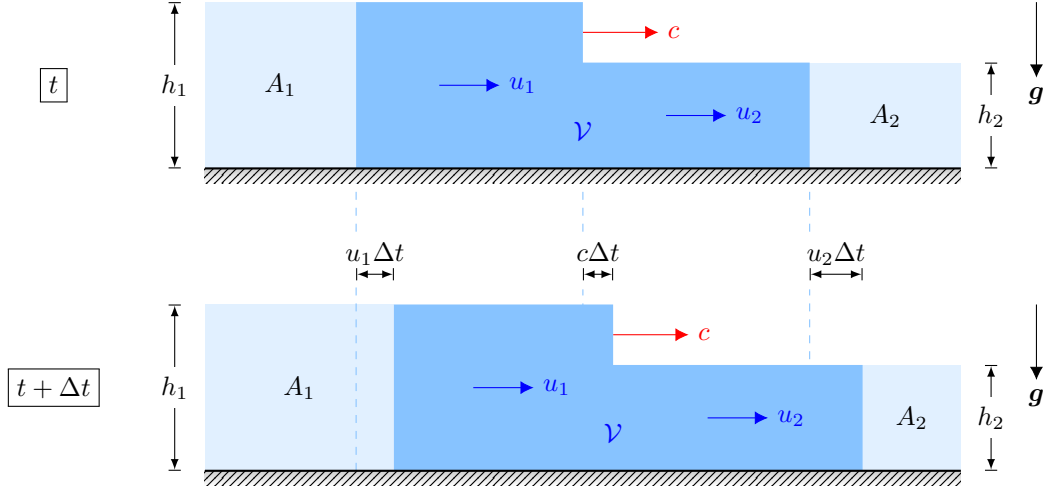
圖 19. t 與 t + \Delta t 的區域變化。
