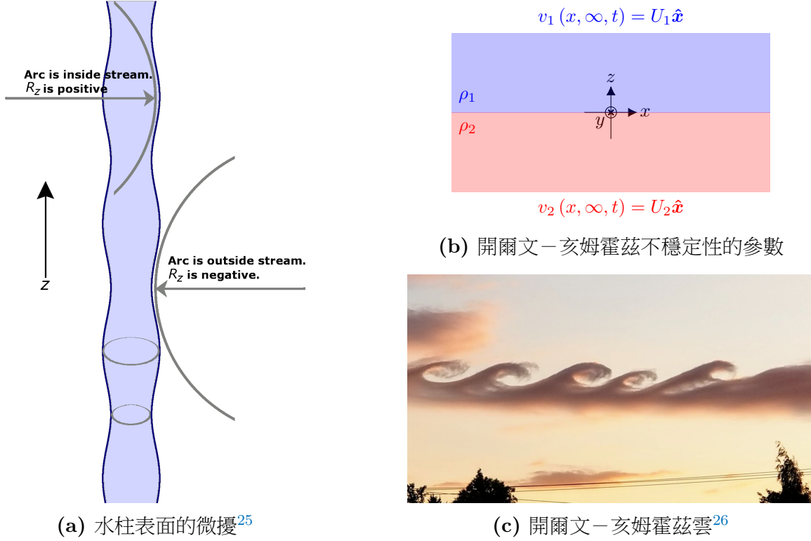
圖 20. 不穩定性之示意圖
