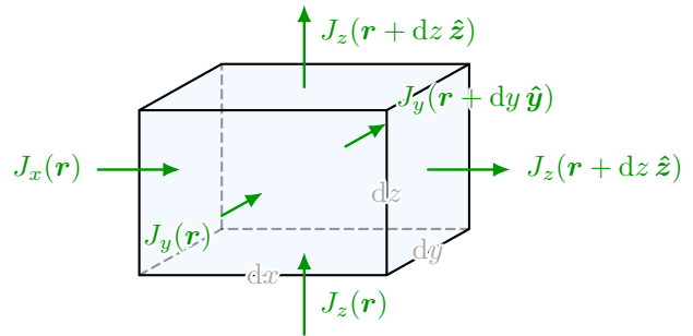
圖 4. 微元的質量流率。 \mathbf{J} = \rho \mathbf{v} 。
