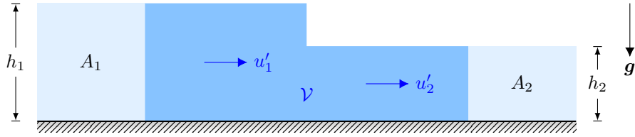
圖 18. 波前坐標系的流速分布。
