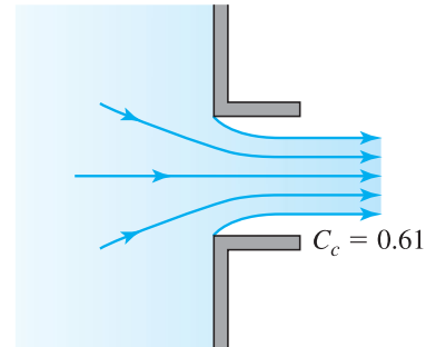
圖 16. 有外壁延伸的開口 [3, p.521]
