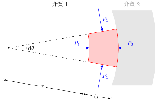
圖 10. 紅色線為環積分路徑。
