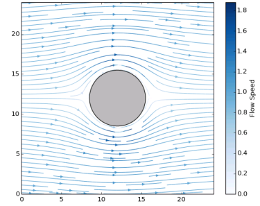
圖 22. 球體所造成的流場 29
