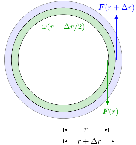
圖 14. 分析二：受力示意圖。
