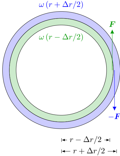
圖 13. 分析一：受力示意圖。
