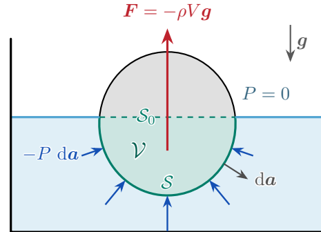
圖 1. 液體壓力的分布及其總合力。
