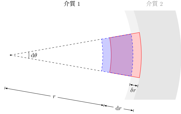
圖 11. 微擾變化示意圖。
