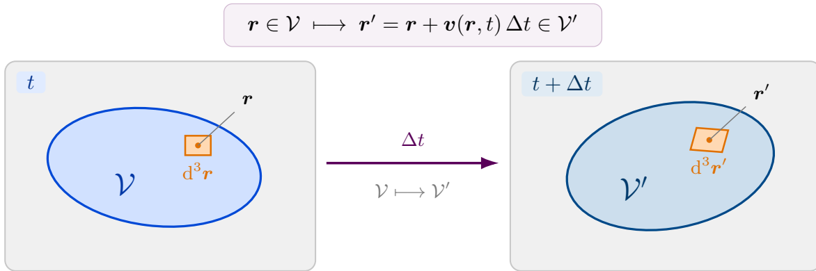
圖 5. \mathcal{V} 中的點與微元經過時間 \Delta t 後映射至 \mathcal{V}' 。
