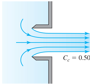
圖 17. 有內壁延伸的開口 [3, p.521]
