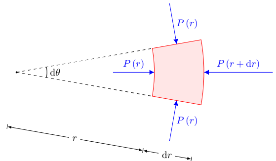
圖 3. 微小質元受力圖
