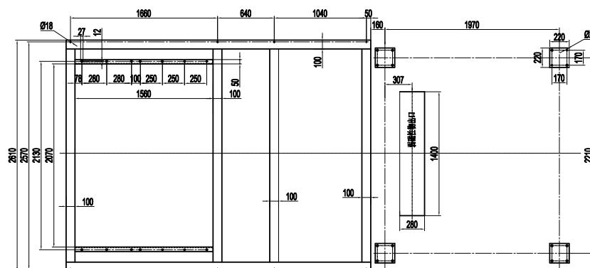
A向底脚视图
