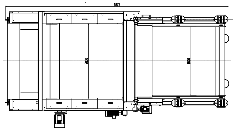
A向底脚视图
