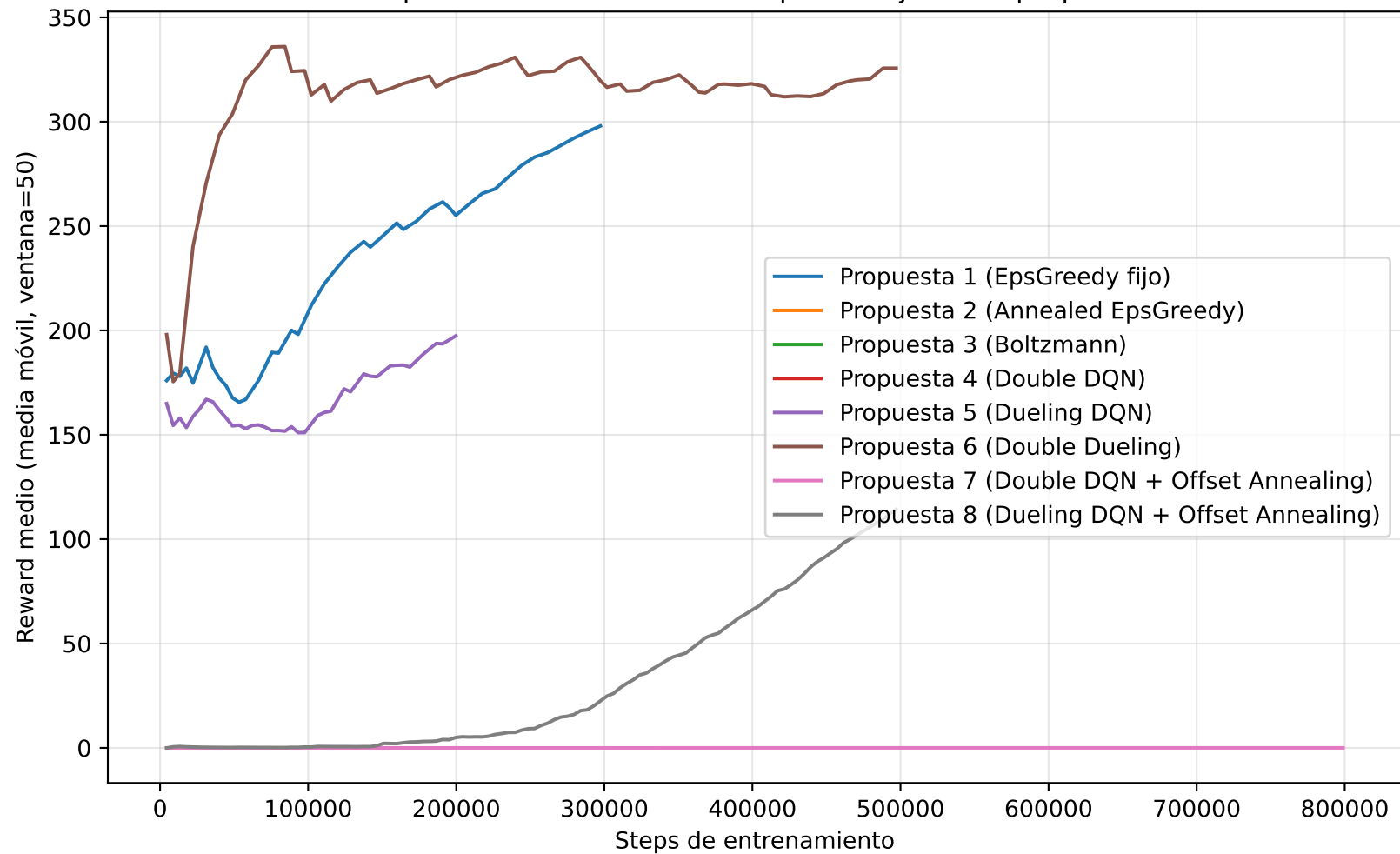
Comparación de velocidad de aprendizaje entre propuestas
