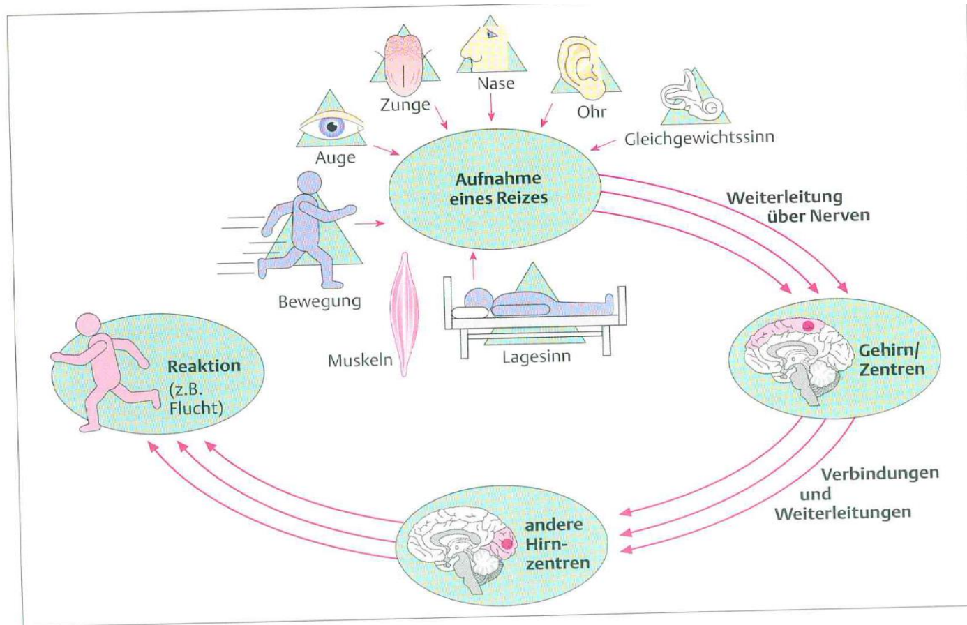
Abb. 1.1 Wahrnehmungsprozess
