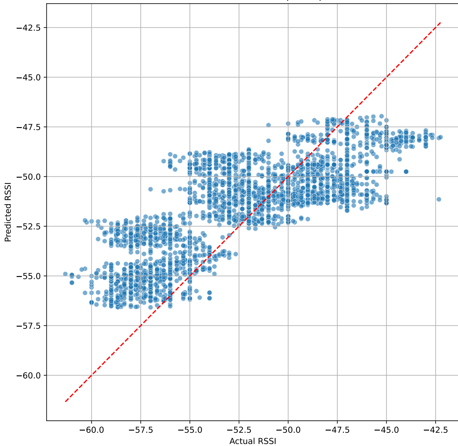
Actual vs Predicted RSSI (Last Step - step 150 \approx 6.0 s)
