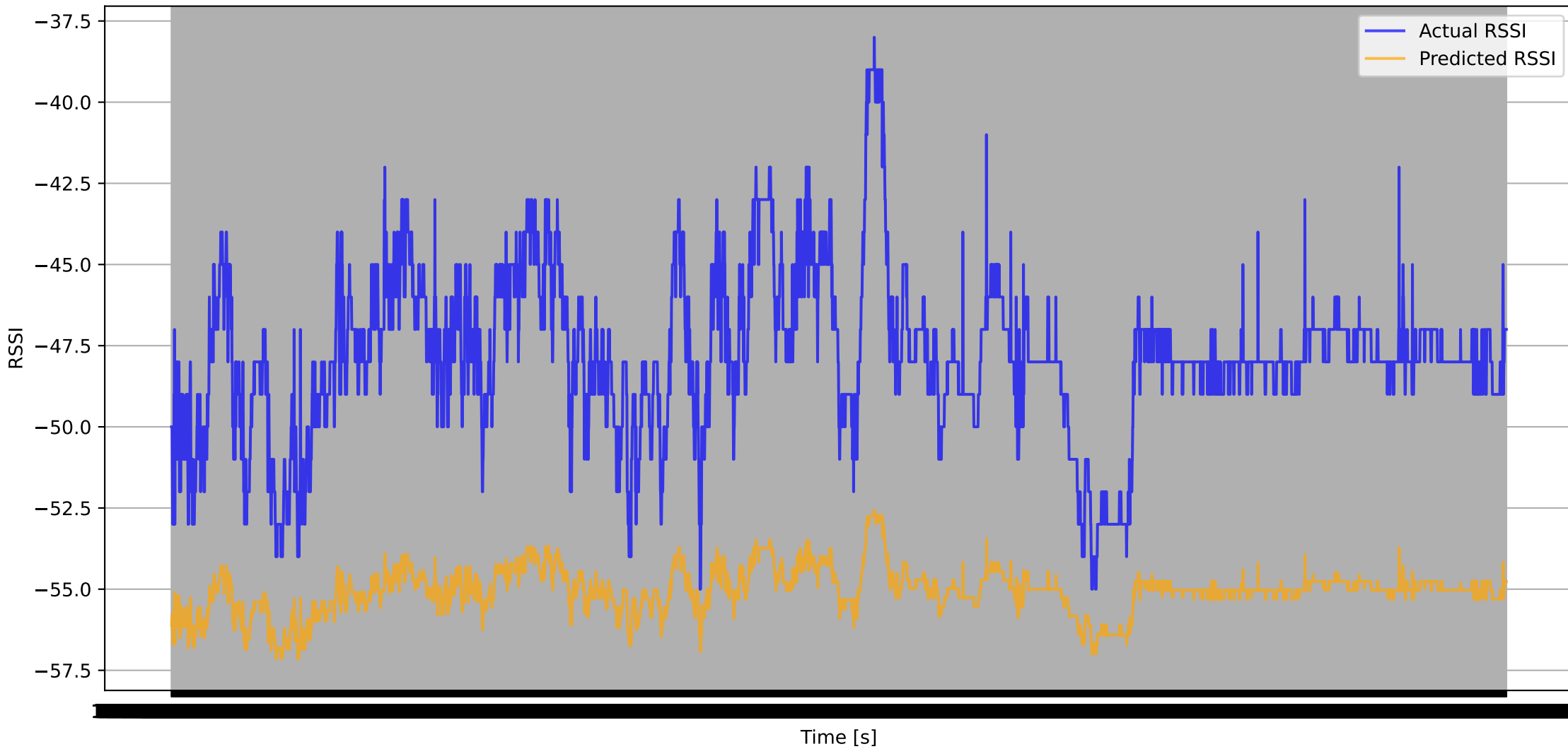
Actual vs Predicted RSSI (First Step)
