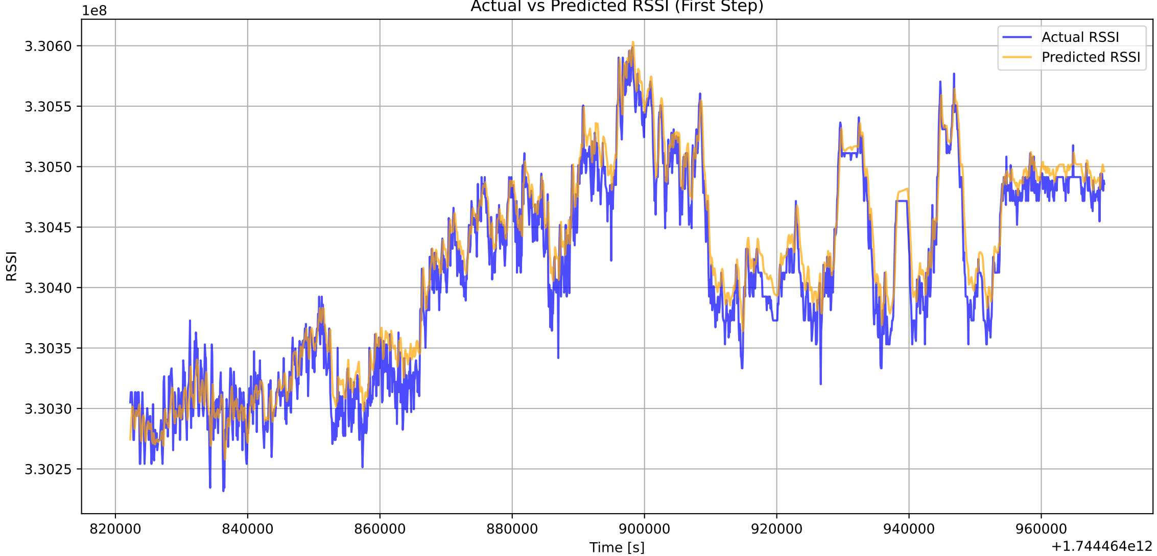
Actual vs Predicted RSSI (First Step)
