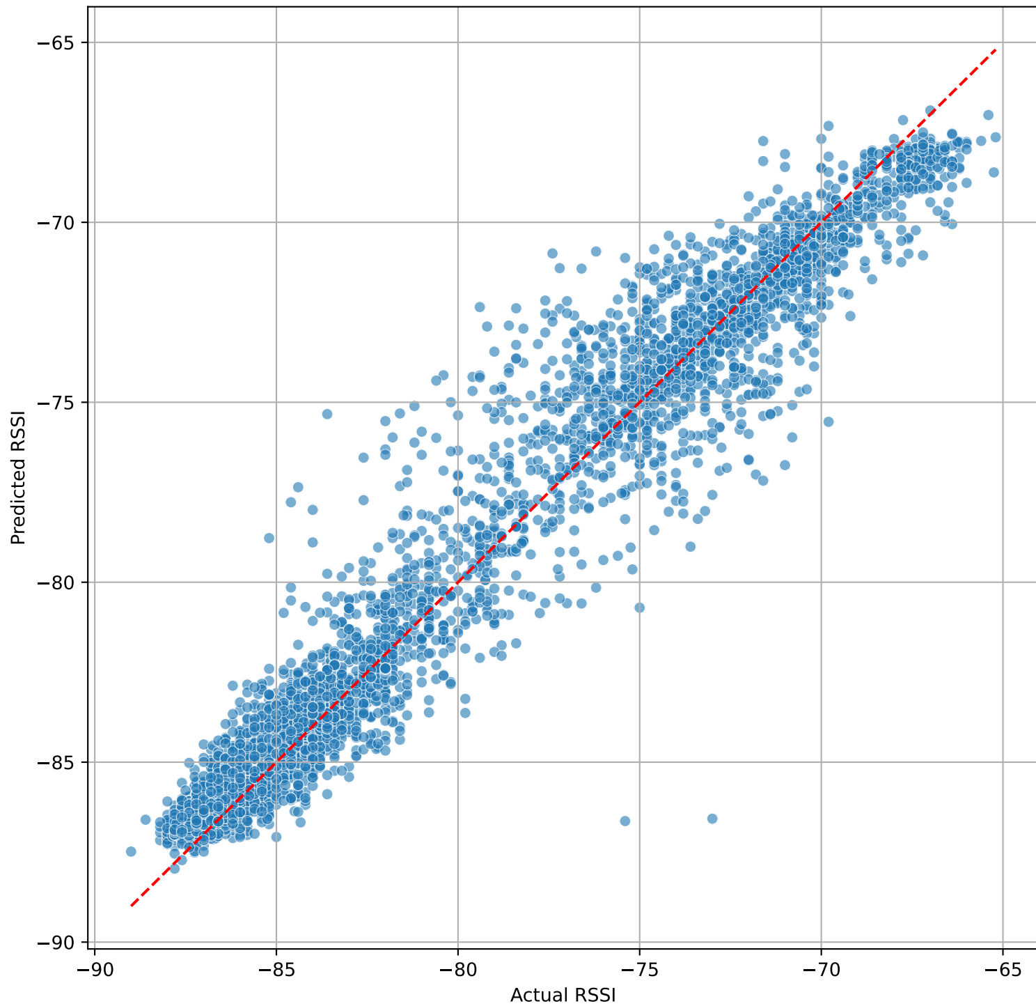
Actual vs Predicted RSSI
