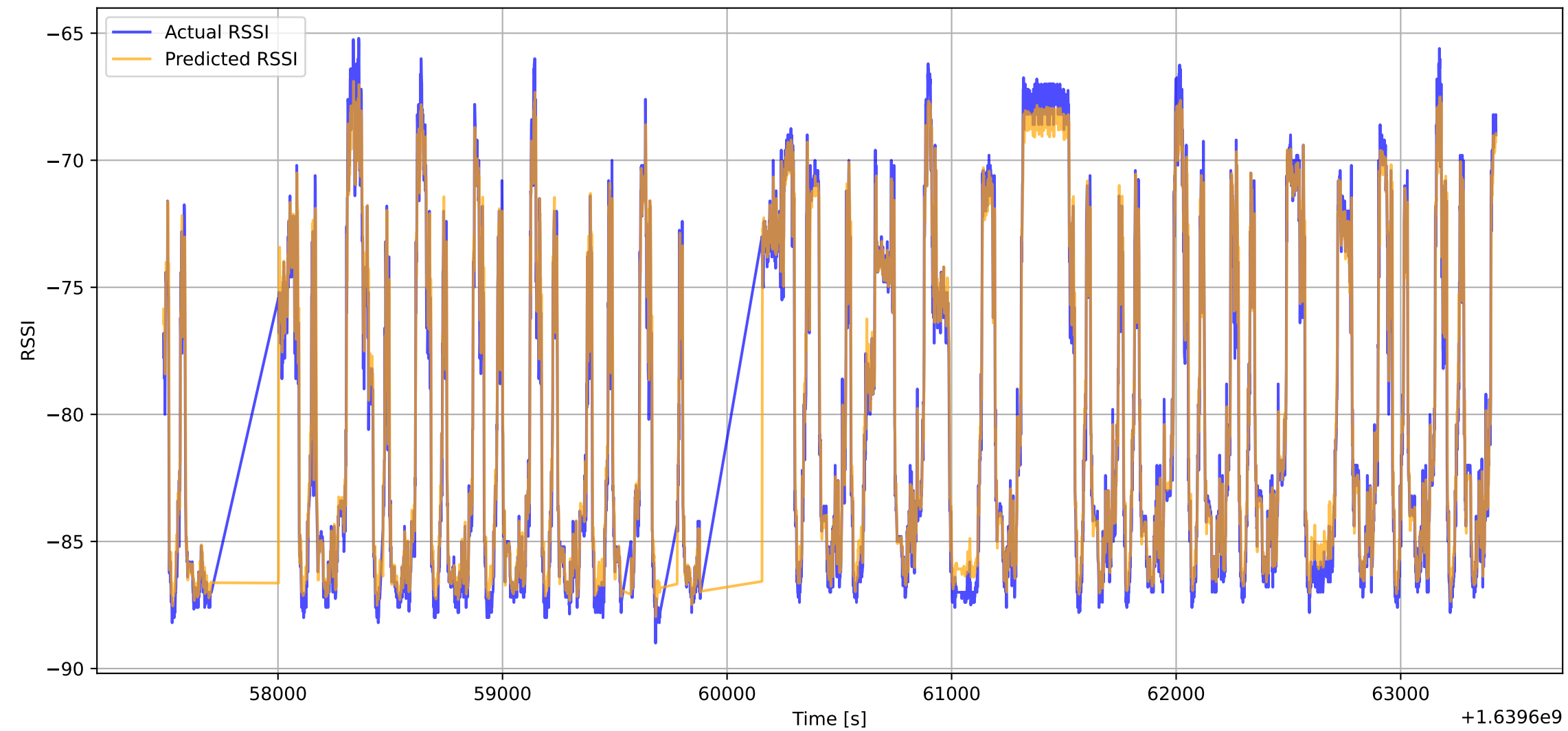
Actual vs Predicted RSSI Over Time
