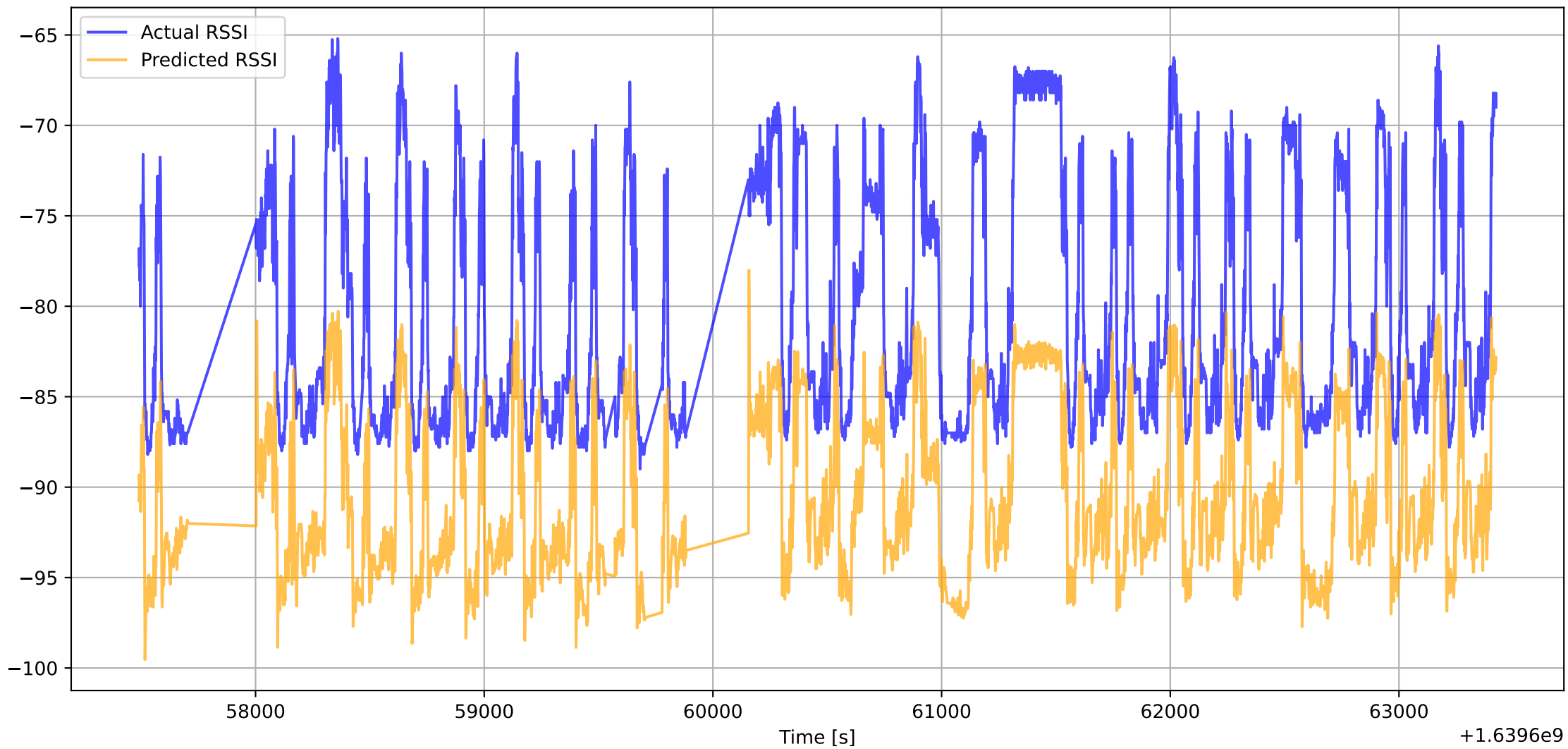
Actual vs Predicted RSSI Over Time
