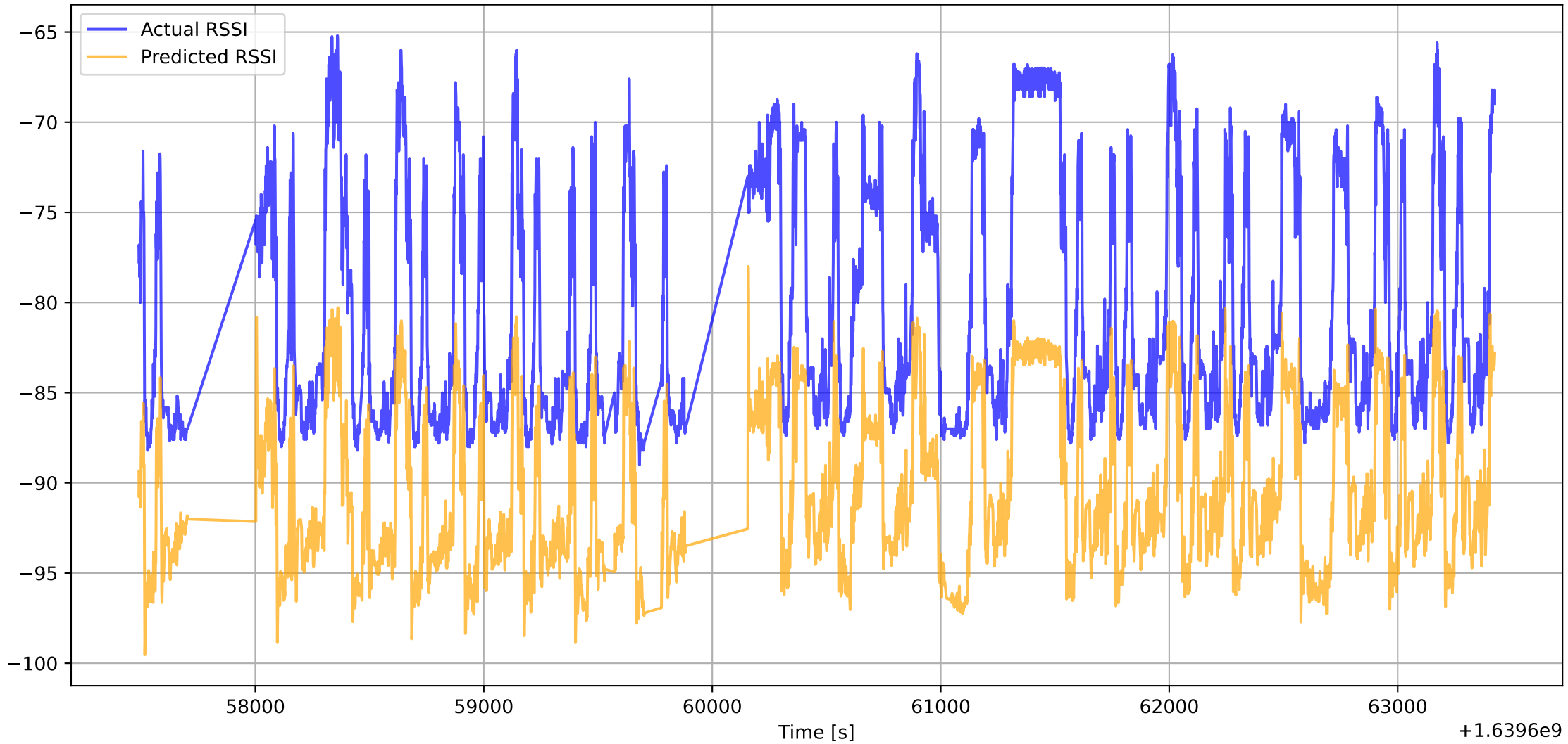
Actual vs Predicted RSSI Over Time
