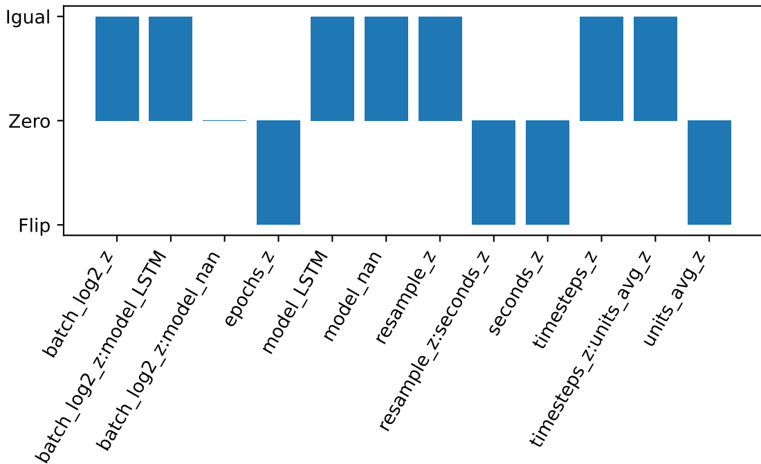
Consistência de sinais dos coeficientes ( A \rightarrow B vs B \rightarrow A )
